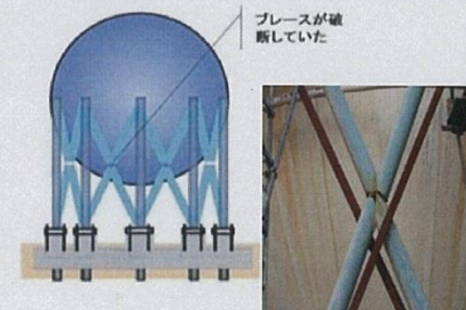
耐震基準の見直しを実施する球形貯槽ブレース
