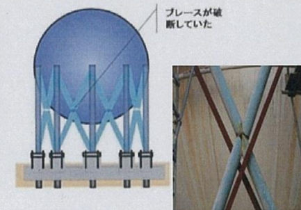
耐震基準の見直しを実施する球形貯槽ブレース
