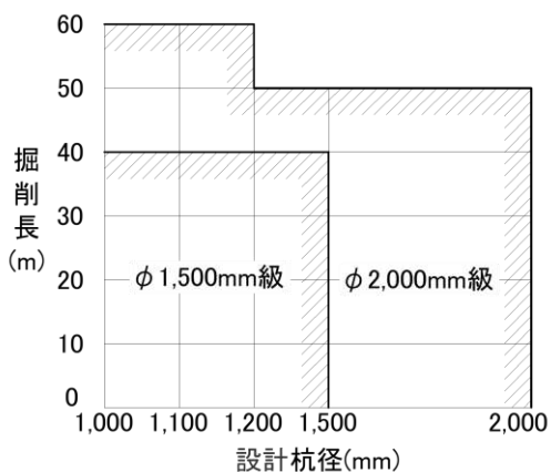
図3-1 掘削機別選定
