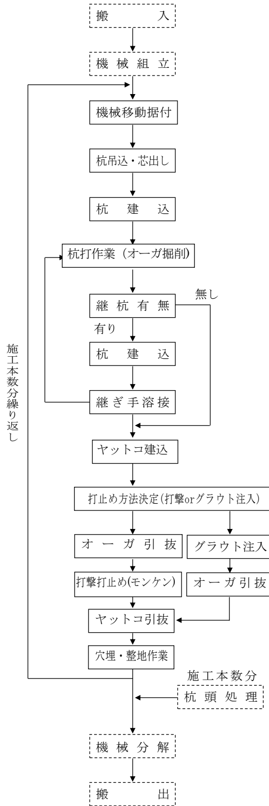
図 2-1 施工フロー
