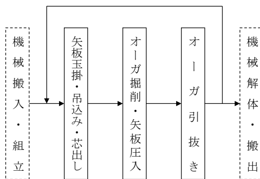
図 2-1 施工フロー
