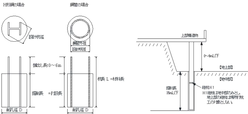
図1-1 施工図
