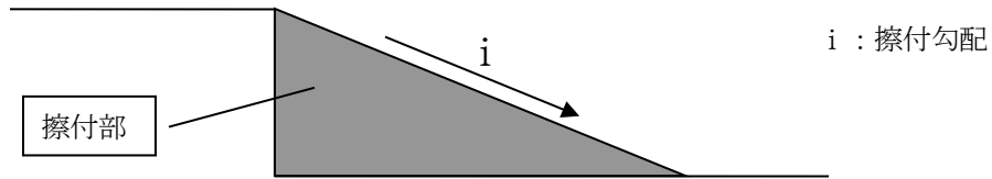
【標準図】
