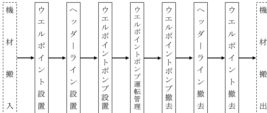
図2-1 施工フロー
