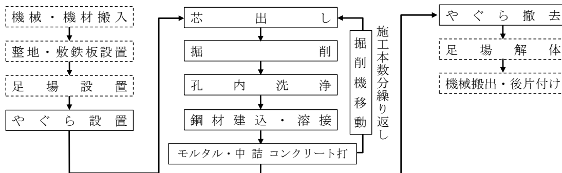
図2-1 施工フロー
