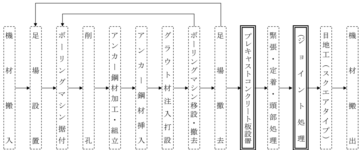
図2-1 施工フロー
