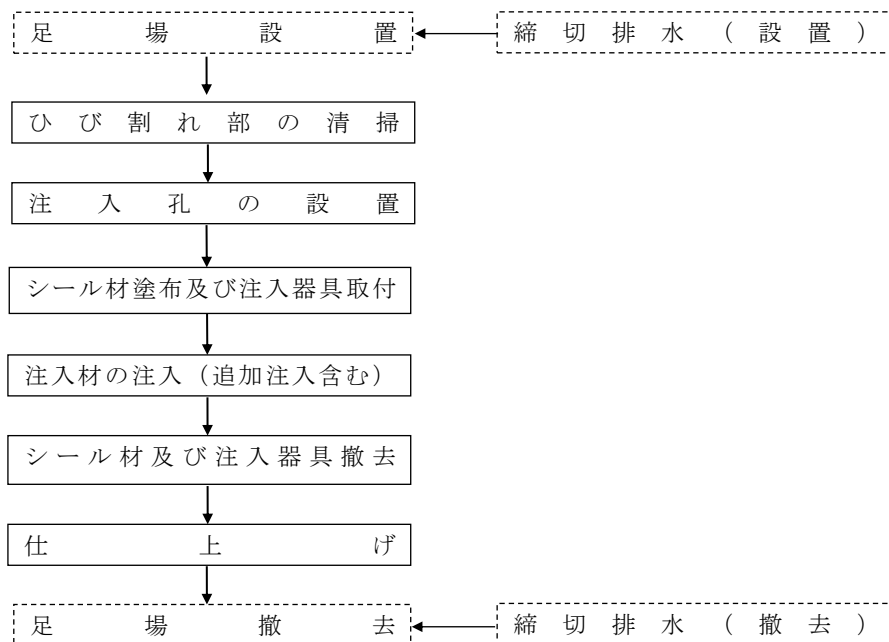
図2-1 施工フロー
