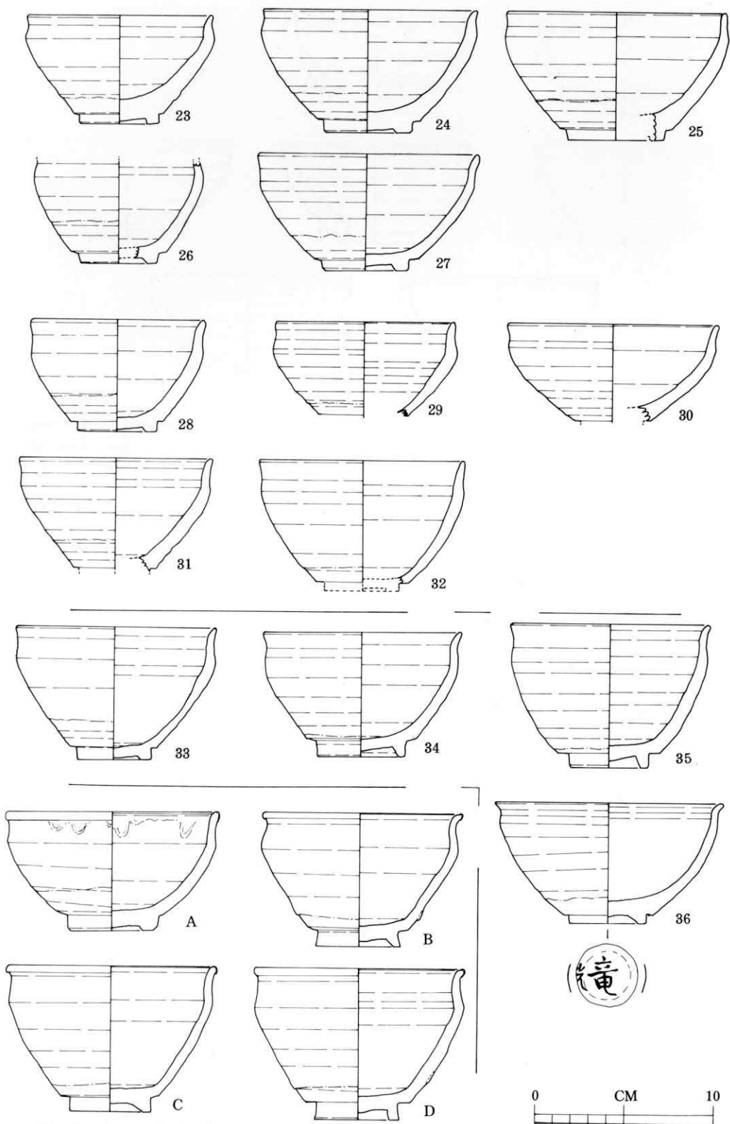
第3図 金谷町上志戸呂古窯出土品(23~32)および同町横岡金谷地区表採品(33~35)、大徳寺什器天目茶碗(36、A~D)実測図；23~25(上志戸呂4類)、26、27(同5類)、28~32(同6類)
