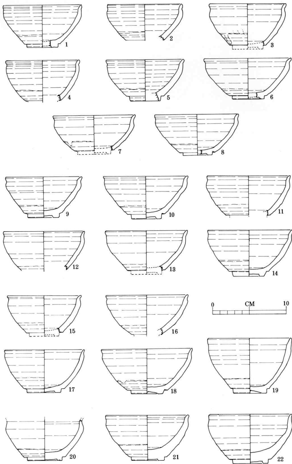
第2図 金谷町上志戸呂古窯出土天目茶碗実測図 1~8 (上志戸呂1類)、9~14 (同2類)、15~19 (同3類)、20~22 (同4類)
