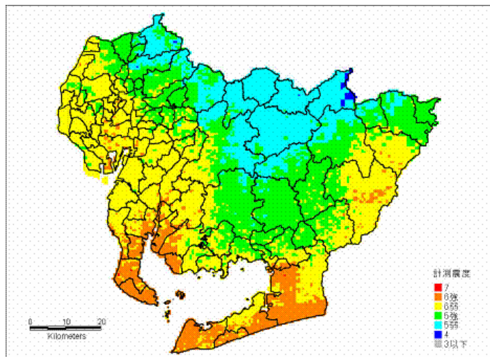
【想定東海・東南海地震連動の予測結果】
