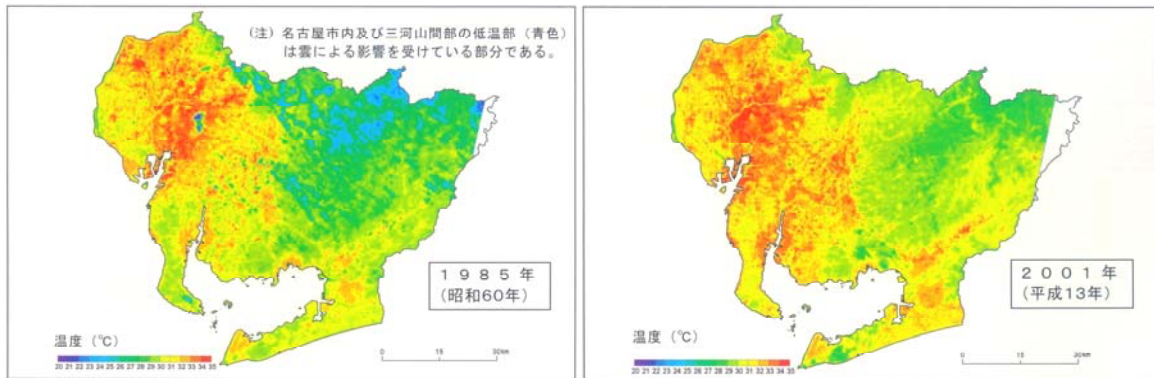
【愛知県内の地表面温度分布の経年比較】
