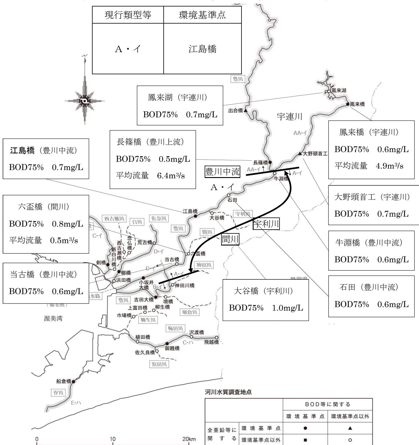
図 3 豊川中流流況図
