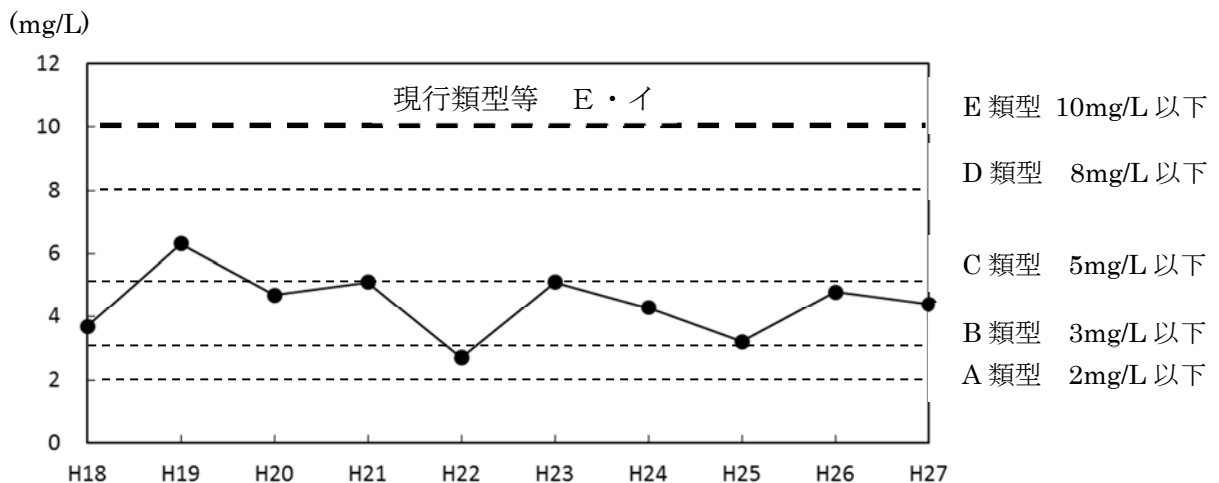
図 1.2 五条川下流域（稲春橋）における BOD(75%値)の状況
