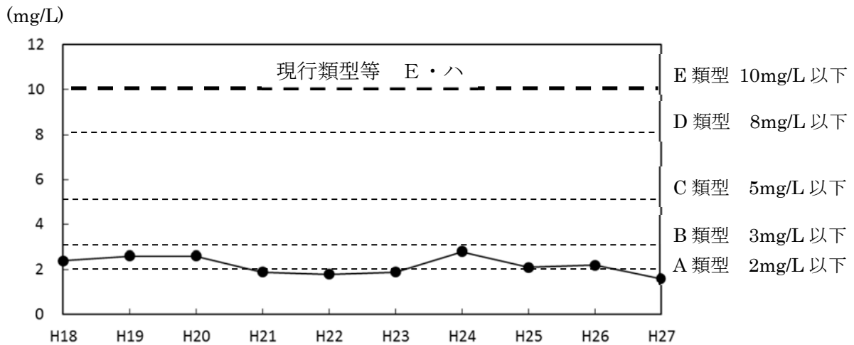
図 1.1 新川下流域（日の出橋）における BOD(75%値)の状況
