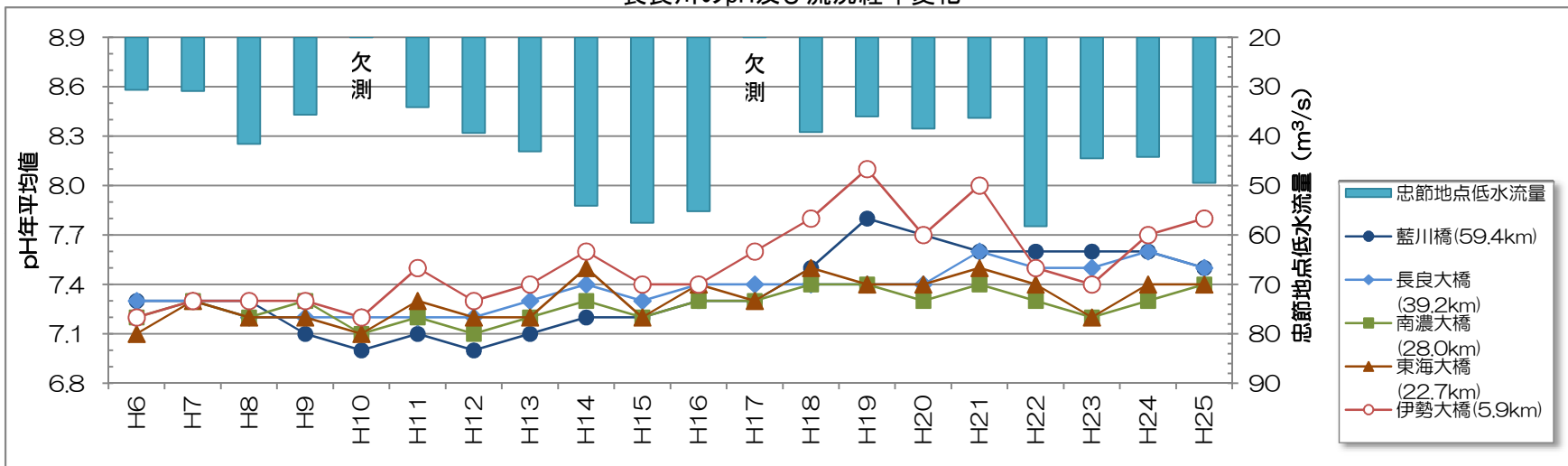
長良川のpH及び流況経年変化
