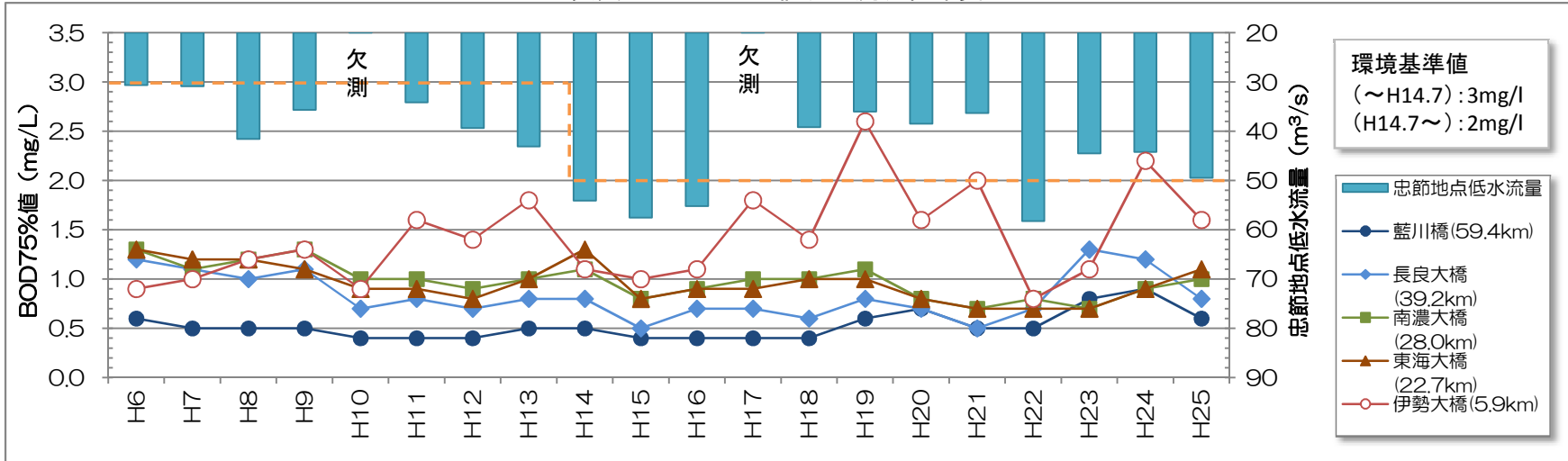
長良川のCOD及び流況経年変化
