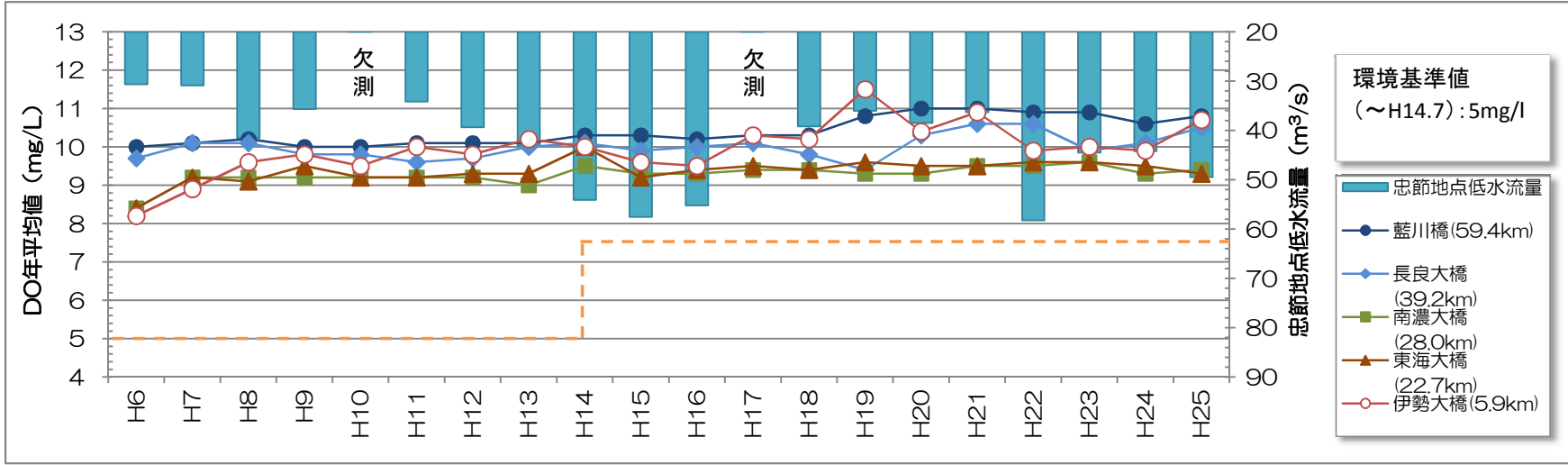
長良川のBOD75%値及び流況経年変化
