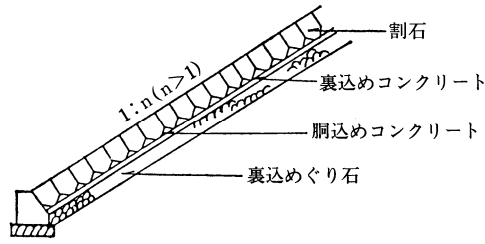
図 5-8 石張工の例
