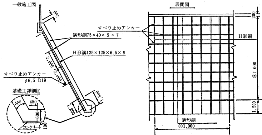
図 5-9 コンクリート張工の例
