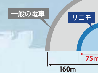
一般の電車では半径160mは必要です。
