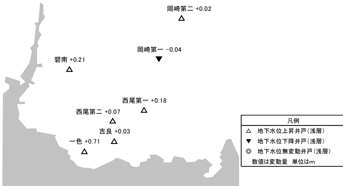
図 2 - 8 西三河浅層の地下水位変動状況 (7井) (平成 27 年と 28 年の平均地下水位比較)
