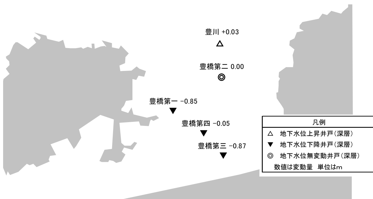
図 2 - 13 東三河深層の地下水位変動状況 (5 井) (平成 27 年と 28 年の平均地下水位比較)
