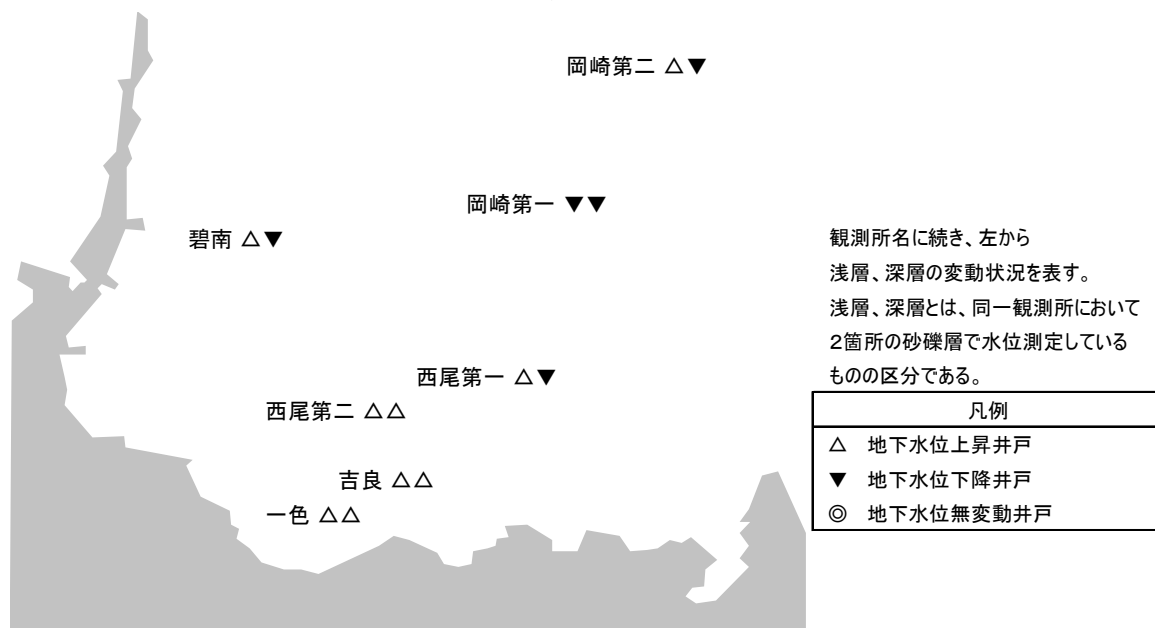
図 2-7 西三河観測井の地下水位変動状況 (平成 27 年と 28 年の平均地下水位比較)
