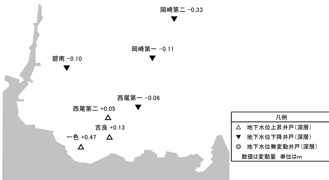
図 2 - 9 西三河深層の地下水位変動状況 (7井) (平成 27 年と 28 年の平均地下水位比較)
