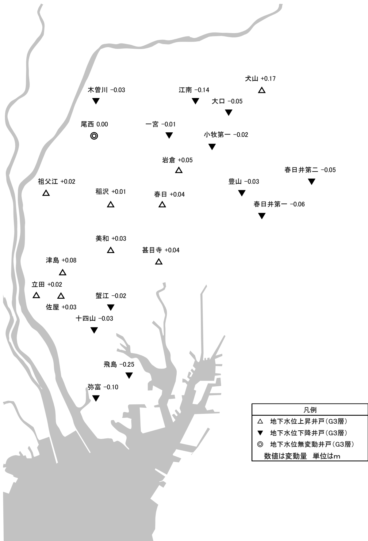
図 2 - 5 観測井G 3層の地下水位変動状況 (23井) (平成 27年と 28年の平均地下水位比較)
