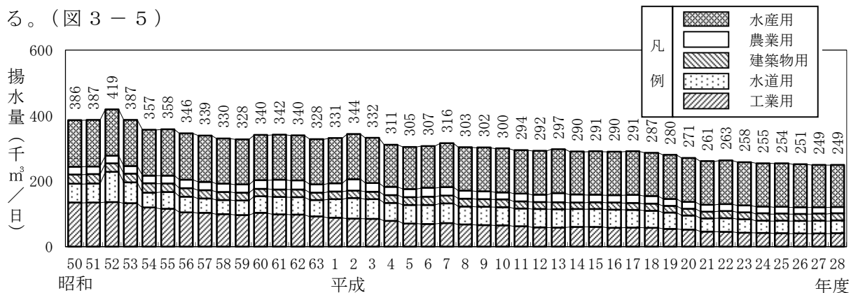
図 3-5 東三河地域地下水揚水量
