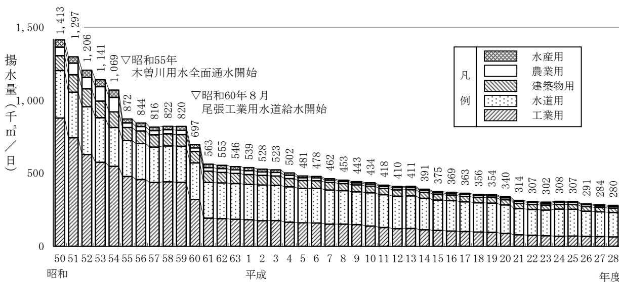
図3-2 尾張地域地下水揚水量(県民の生活環境の保全等に関する条例の規制区域19市町村)
