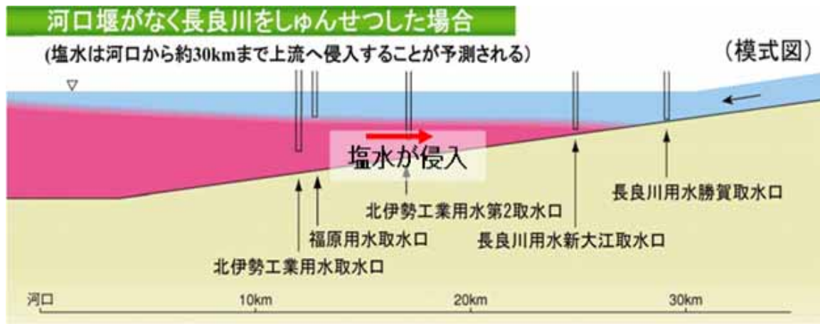
図 4 - 1 0 浚渫による塩水の遡上
