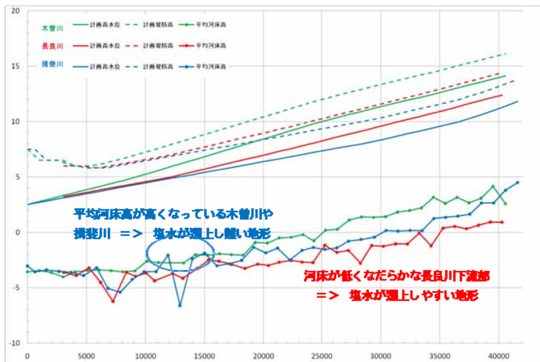
図4-12 木曽川、長良川、揖斐川の河床縦断形状の比較
