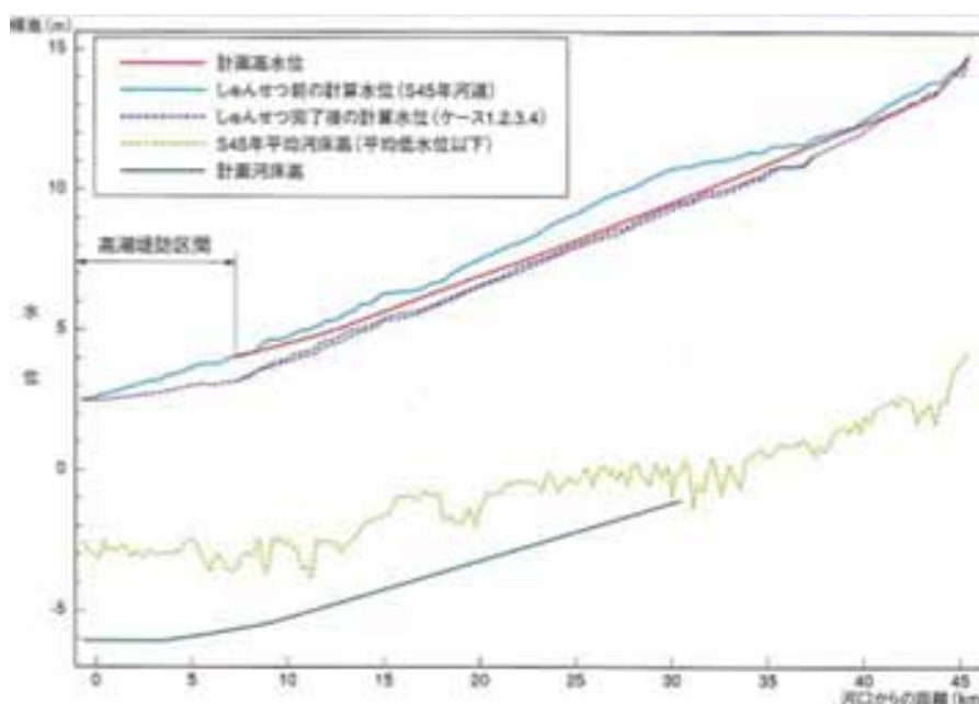
図4-9 浚渫前後の水位比較
