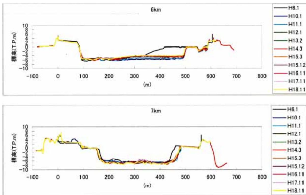
図 2 - 1 3 6km および 7km 地点の河床横断形状の変化
