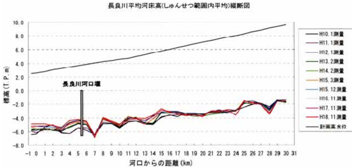
図 4 - 5 長良川平均河床縦断面図
