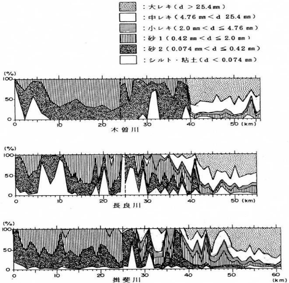
図2-9 粒度分布の縦断変化
