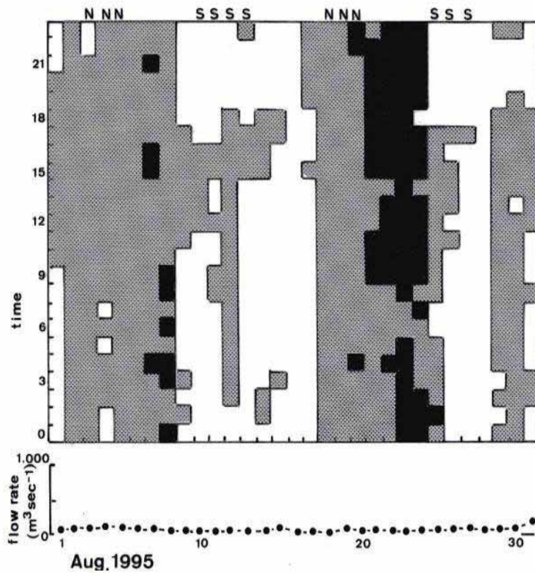
図 2 - 5 河口堰下流の溶存酸素濃度
