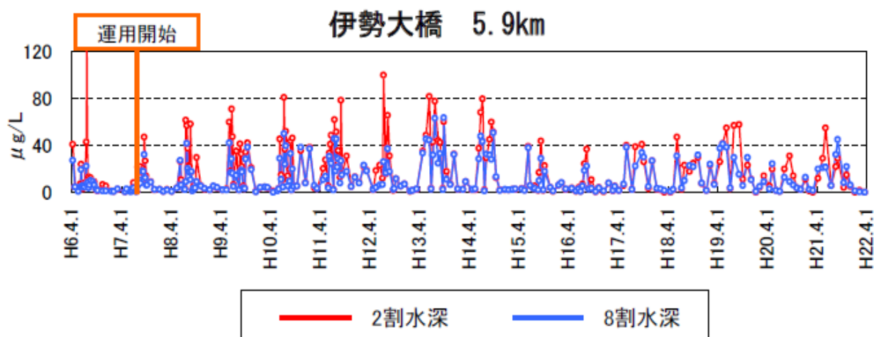
図 2-3 事業者測定による藻類発生量(クロロフィル a 濃度)の経年変化
