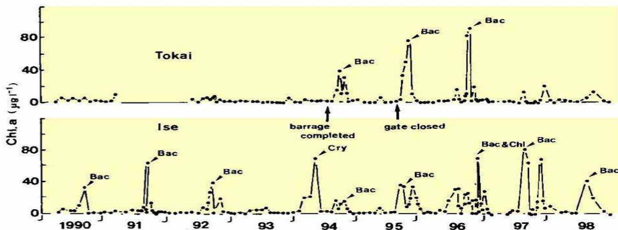
図 2-2 藻類発生量(クロロフィル a 濃度)の経年変化
