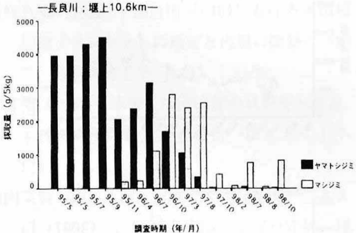
図2-10 ヤマトシジミとマシジミの採取量の推移
