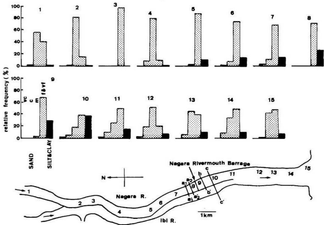
図 2 - 7 長良川河口堰付近の河床堆積物粒度組成
