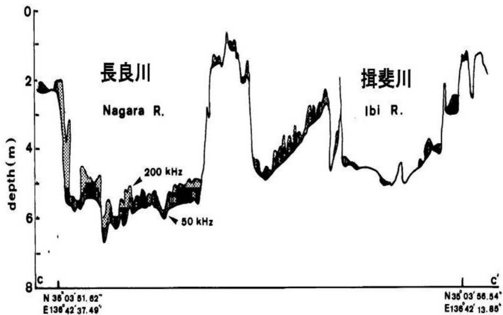
図 2 - 8 音波探査による堆積物厚調査結果
