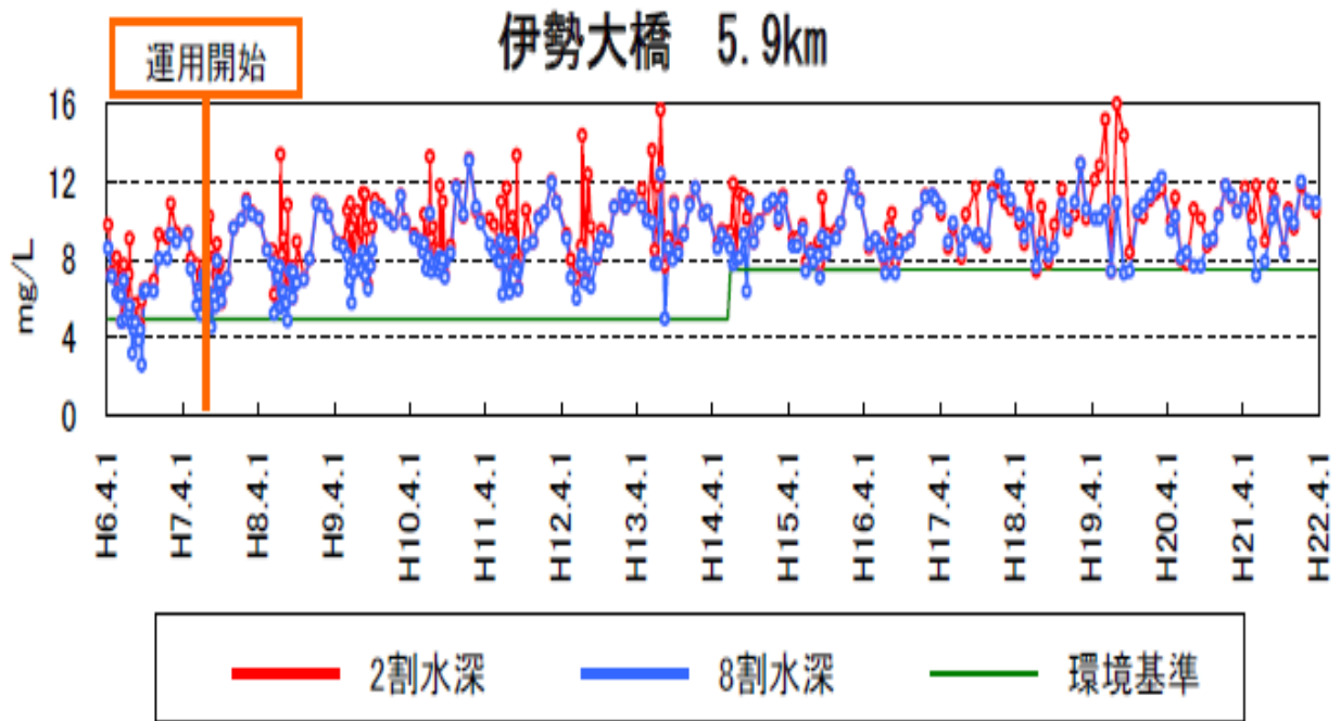
図 2 - 4 事業者測定による DO 測定結果
