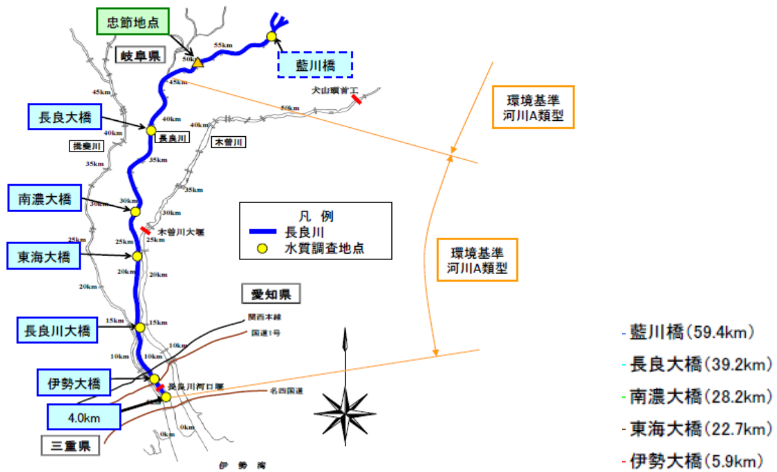
図 2 - 1 事業者の水質調査地点
