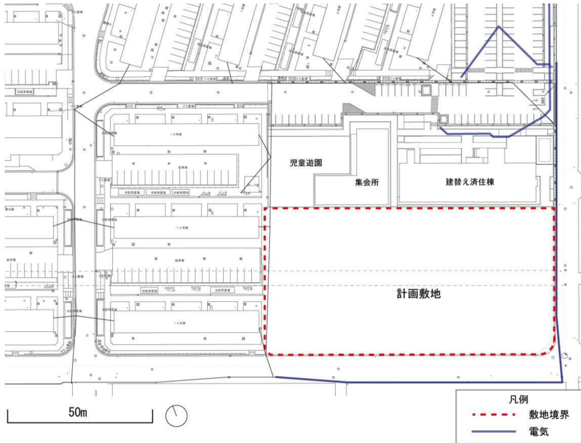
電力供給線
