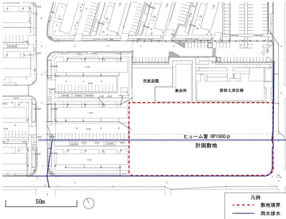
雨水（下水道）
