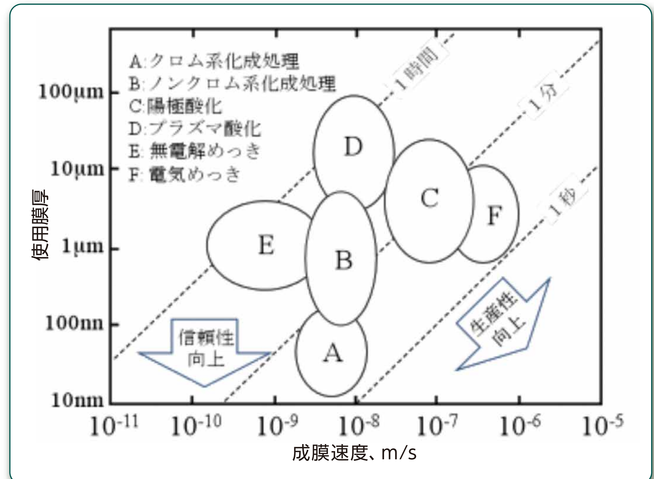
図1 Mgの湿式表面処理の膜厚と作業速度
