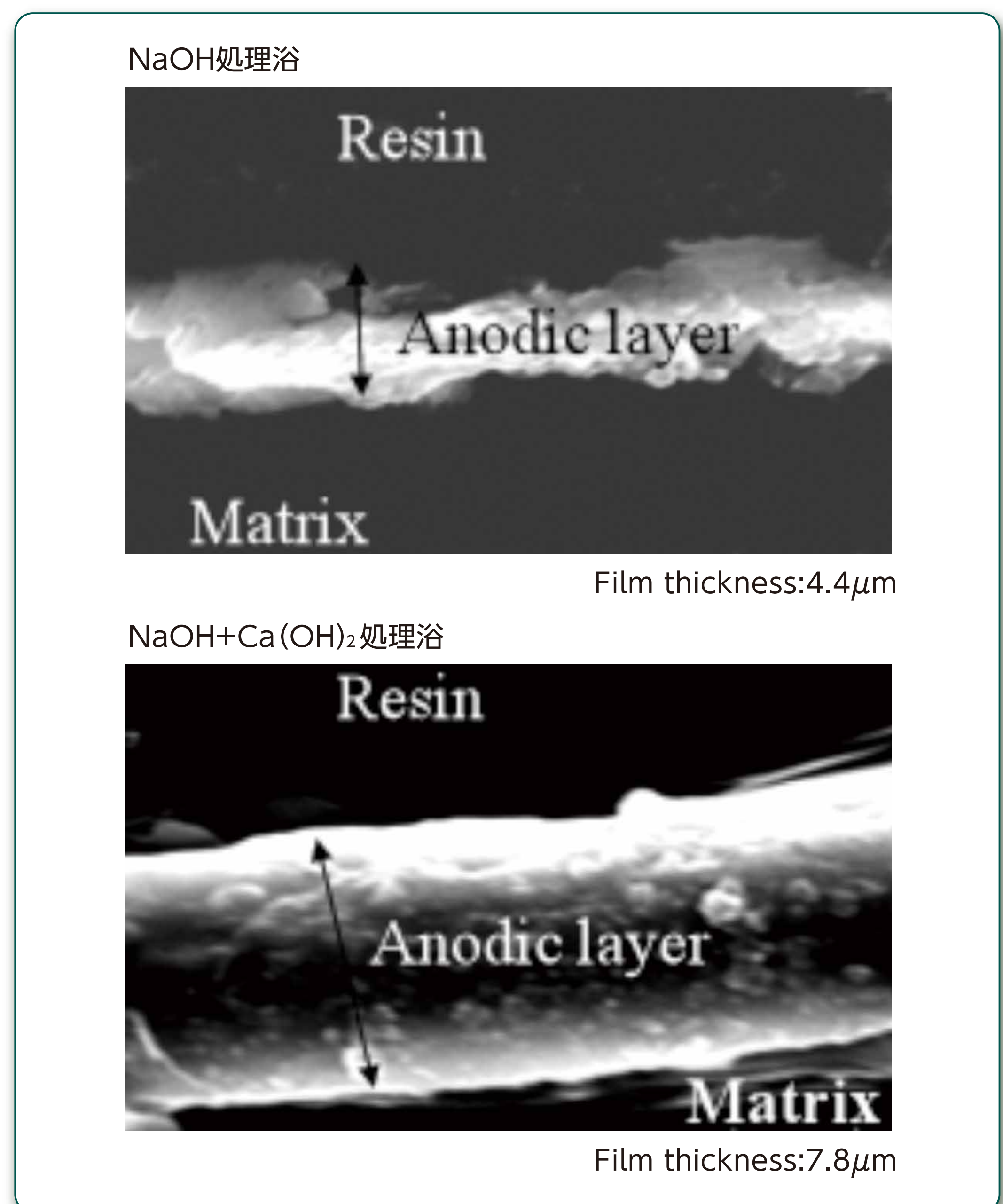
図2 カルシウムによるMg合金の陽極酸化膜の特性向上
