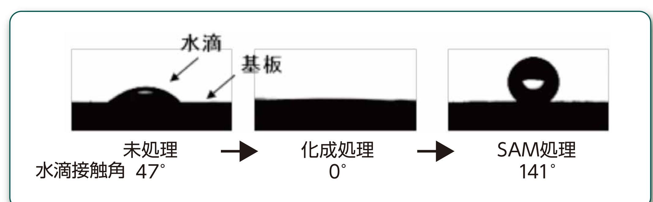
図3 Mg合金のSAM処理による超撥水性の発現
