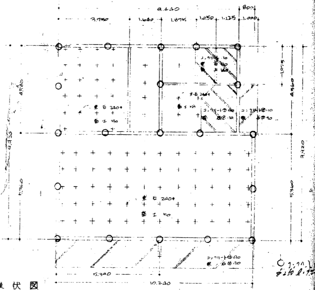
多线伏图
