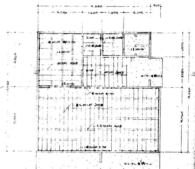
床伏图
