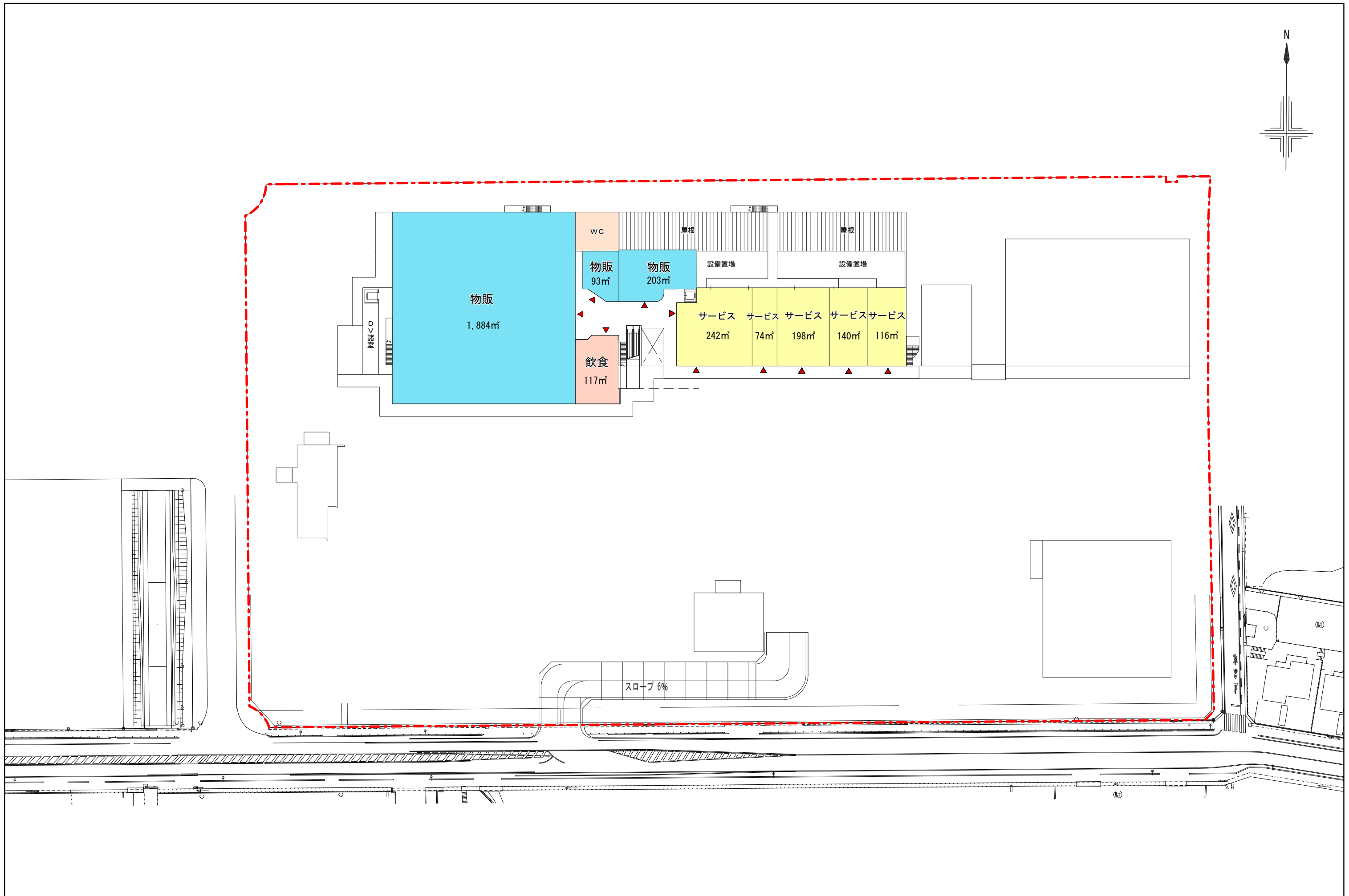
図面 4 2階平面図 (S=1/800)
