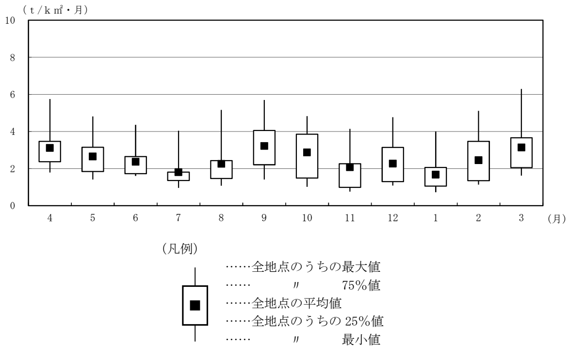
図8-2 降下ばいじん量（平成25年度）の経月変化
