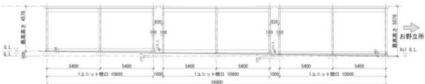
正面図
