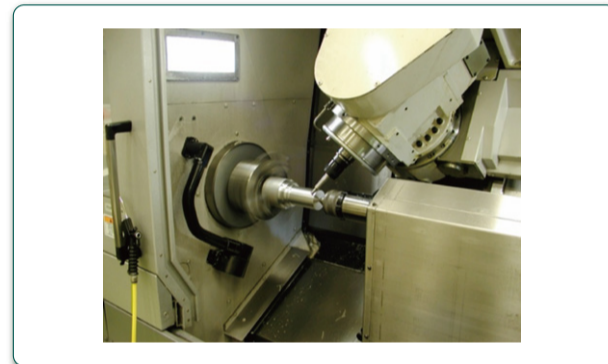
図2 複合加工機によるロータリ切削
