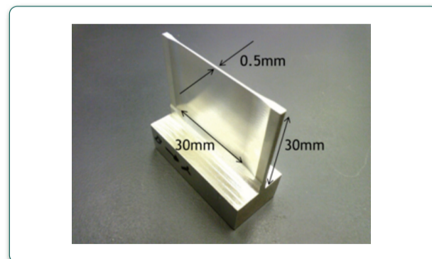
図4 薄肉立壁加工
