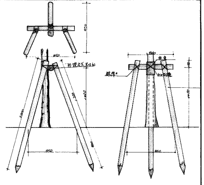
円型トランジ詳細図 1/20
