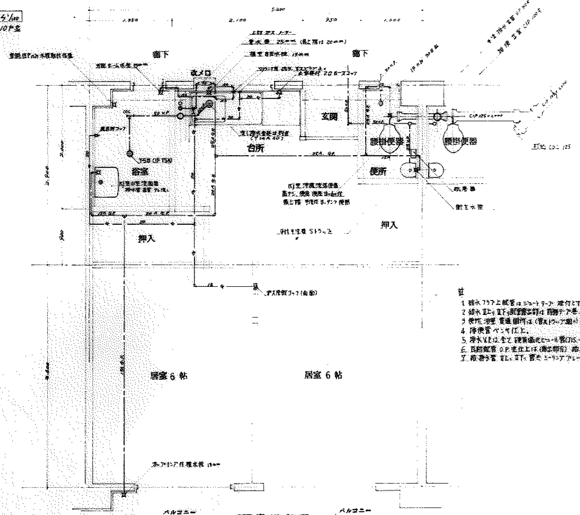
配管詳細図 5/100 68-4N-2DK-1
