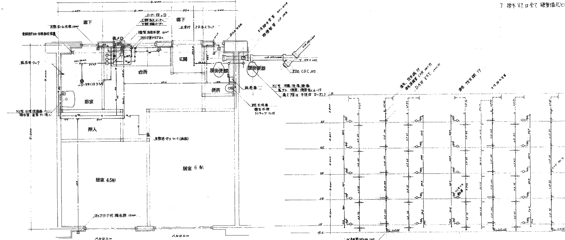
平面配管詳細図 5/100 6B-5N-2H-2
