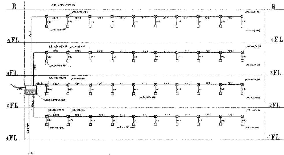
电话配管系统图
