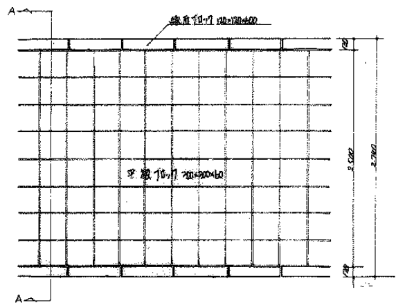
コンクリート詳細図 1/20
