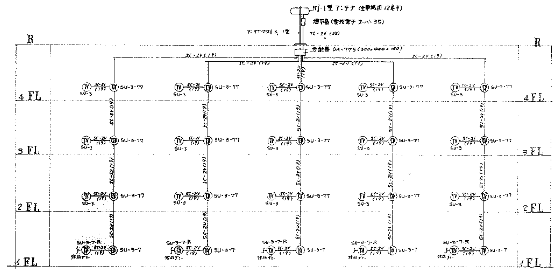
TV集合7寸配管系统图
