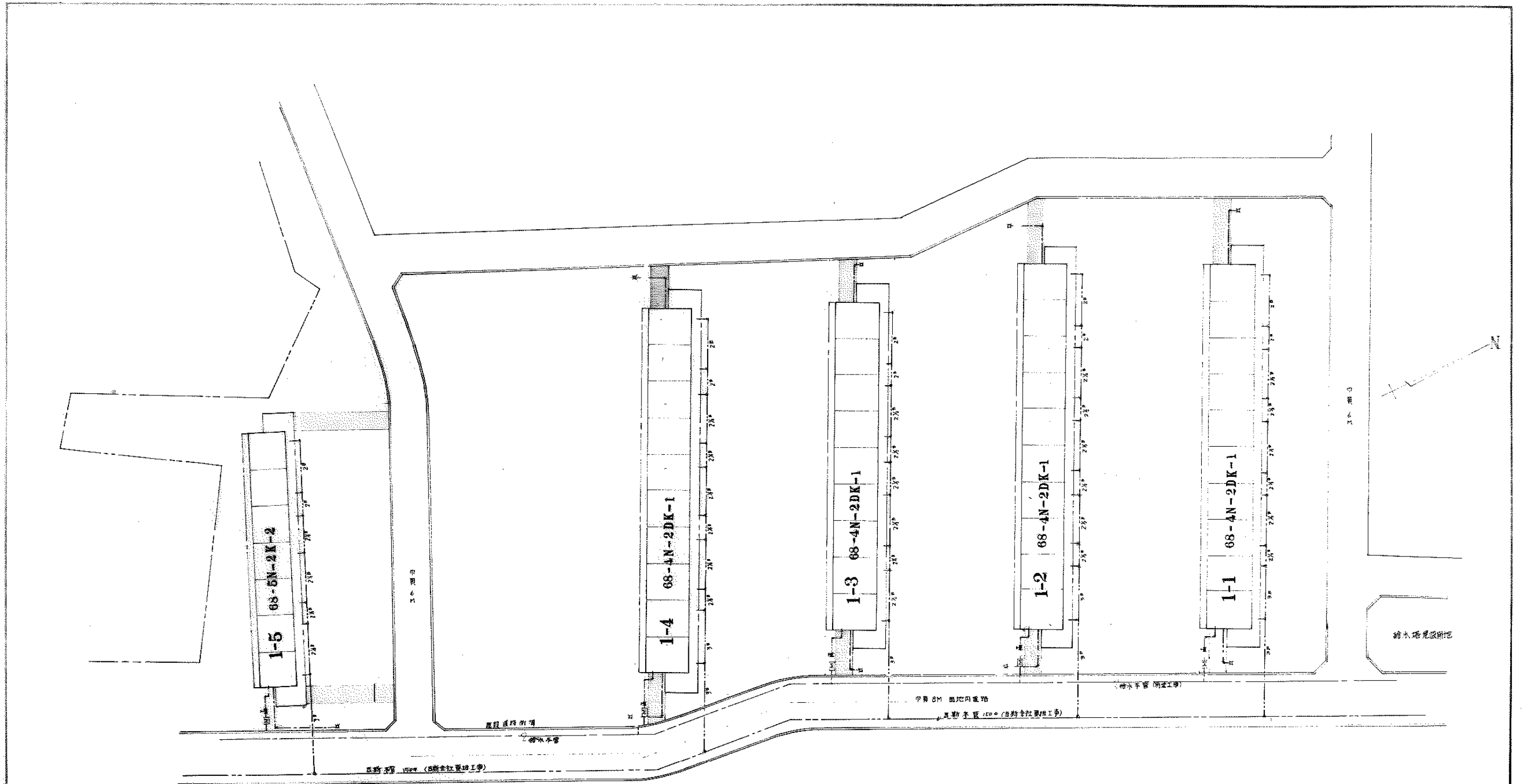
屋外瓦斯配管图 1:500
