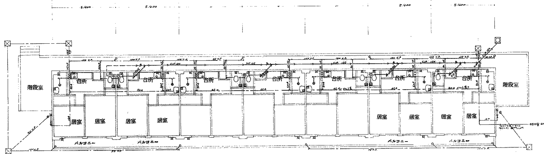
配管平面図 5/100 6B-5N-2H-2型
