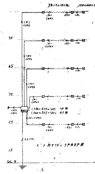
電話配線系統図
