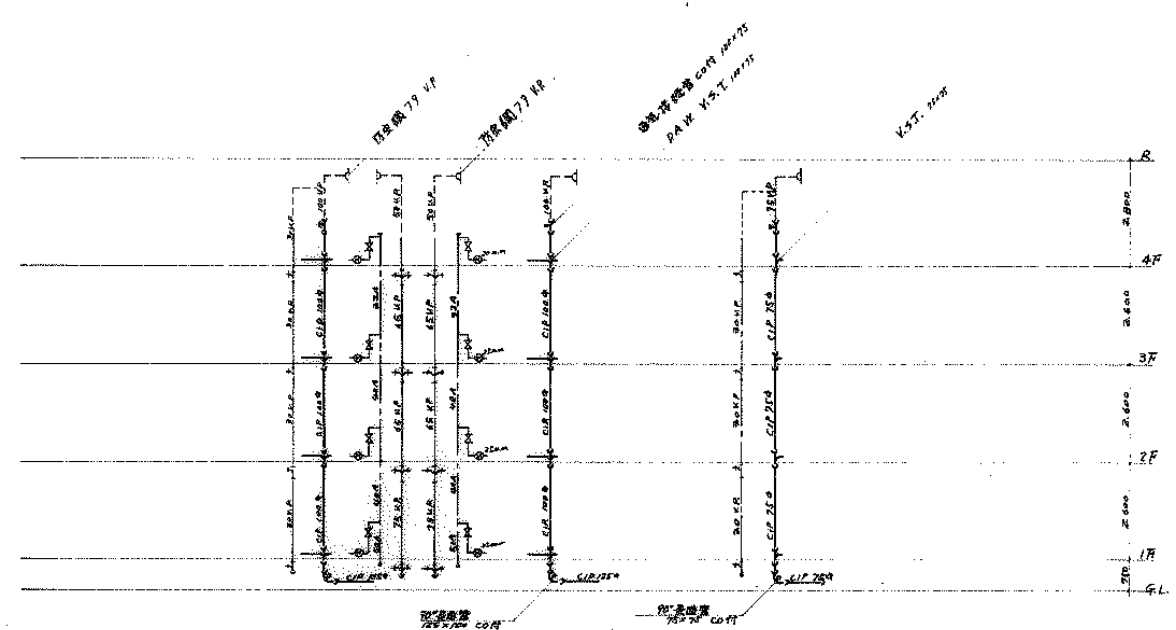
縦管系統図
