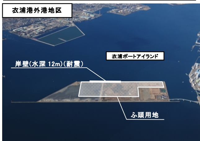
バルク貨物の集約化や船舶の大型化に対応するとともに、大規模地震時には、緊急物資の受入拠点としての役割を担う、水深12mの耐震強化岸壁を整備
