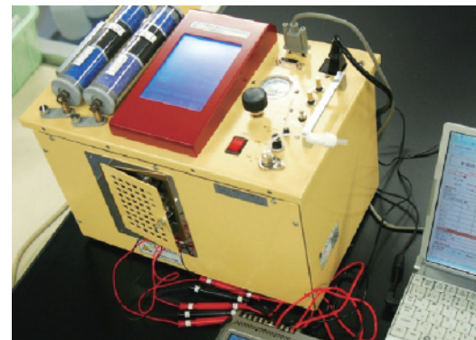
GCと半導体ガスセンサを搭載した試作機
