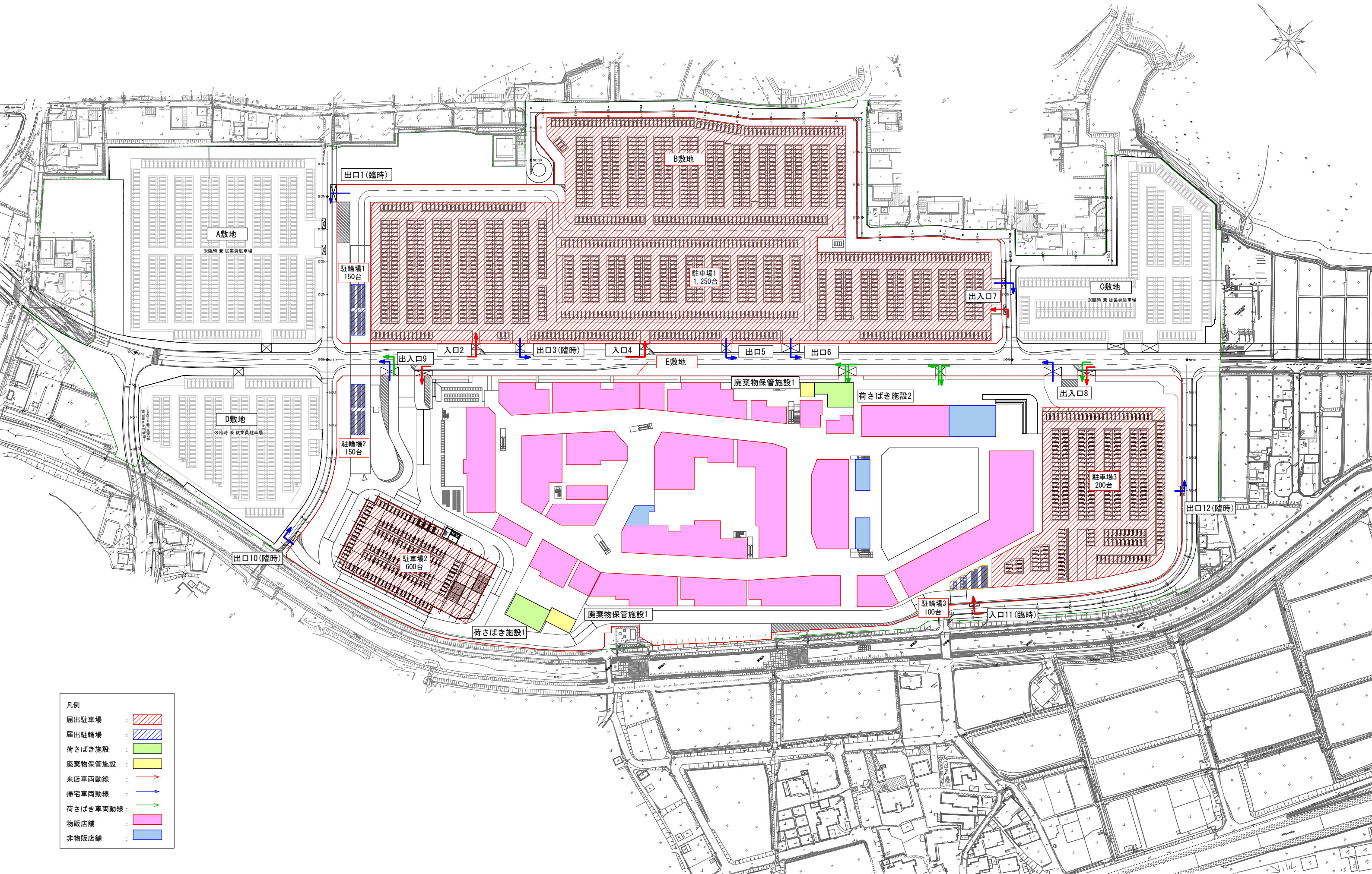
図4 建物配置図 兼 1階平面図 (S=1/2000)
