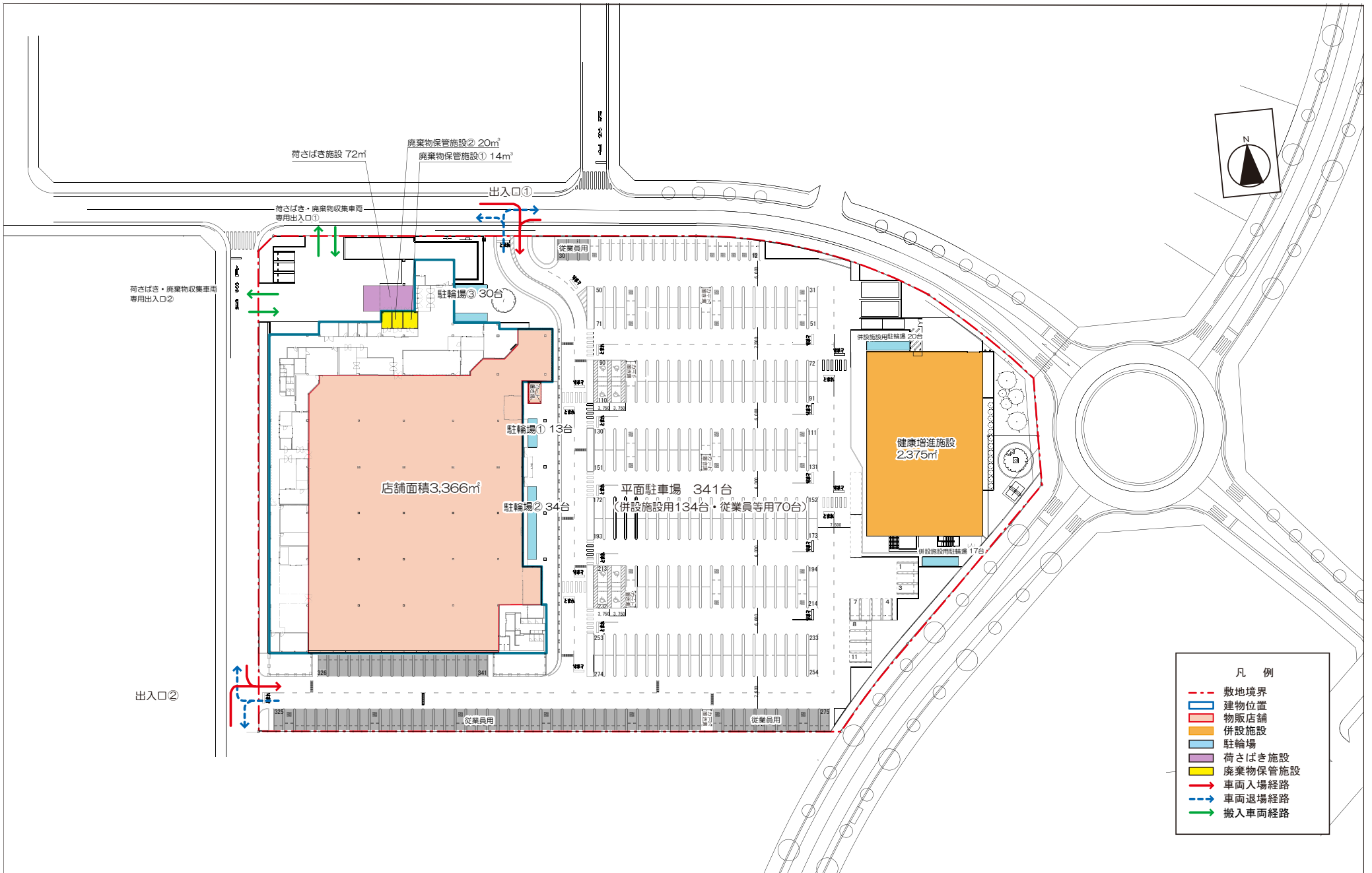
図面3 変更前建物配置図兼1階平面図 (S=1/800)
