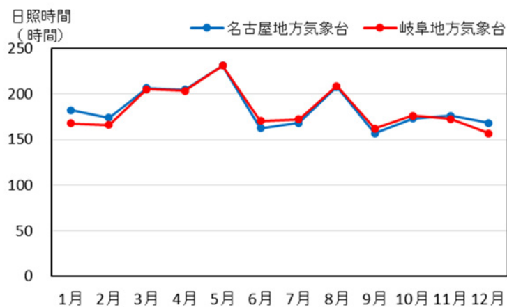
図 4-1-2 月別気象概況（平成 24 年～令和 3 年）
