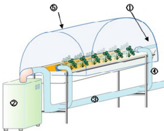
図1 短日・スポット夜冷処理システムの概要 小さな穴をあけたダクト、スポットクーラー、冷気を に送るためのダクト、遮光トンネル
