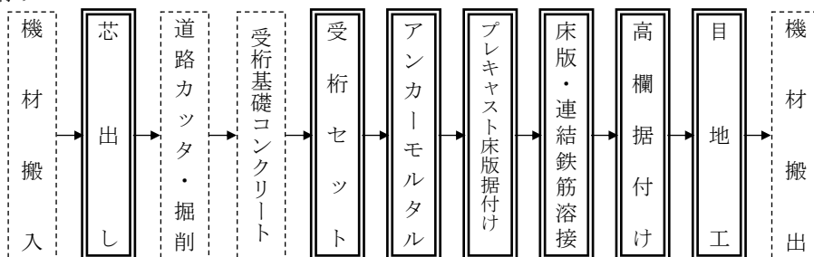
図2-2 施工フロー
