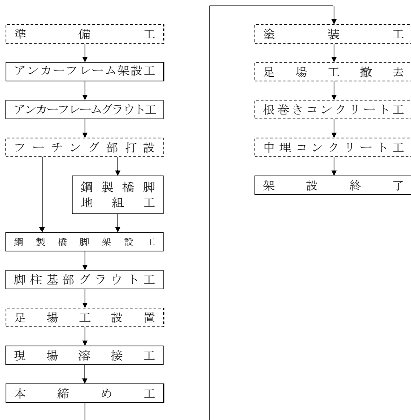
図2-1 施工フロー
