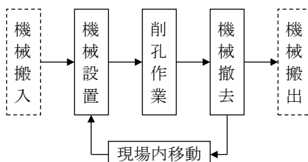
図 2-1 施工フロー
