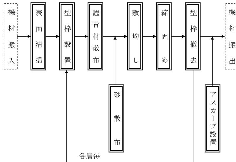
図2-1 施工フロー
