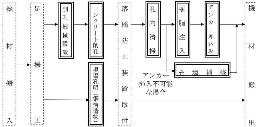
図2-1 施工フロー
