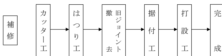
図 4-1 施工フロー(鋼フィンガージョイント等)
