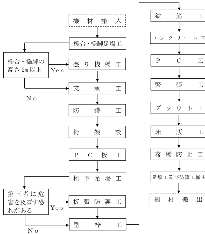
図 2-2 PCコンボ桁 施工フロー
