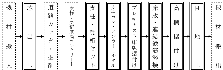
図2-1 施工フロー
