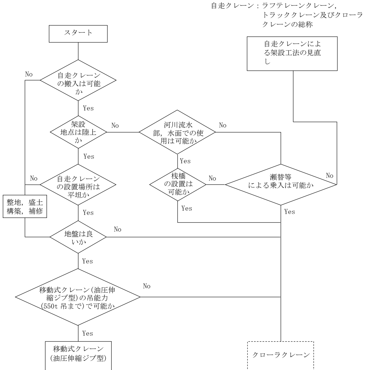
図 18-1 機種選定図
