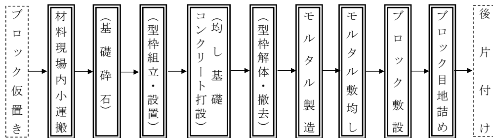
図2-1 施工フロー
