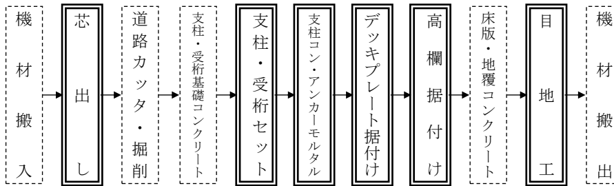
図2-4 施工フロー
