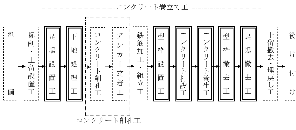
図2-1 施工フロー
