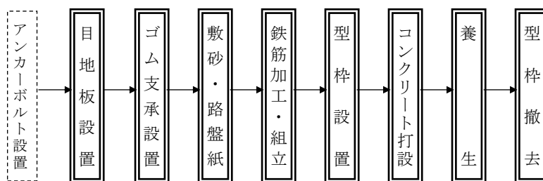
図 2-1 施工フロー
