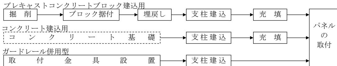
図2-1 施工フロー
