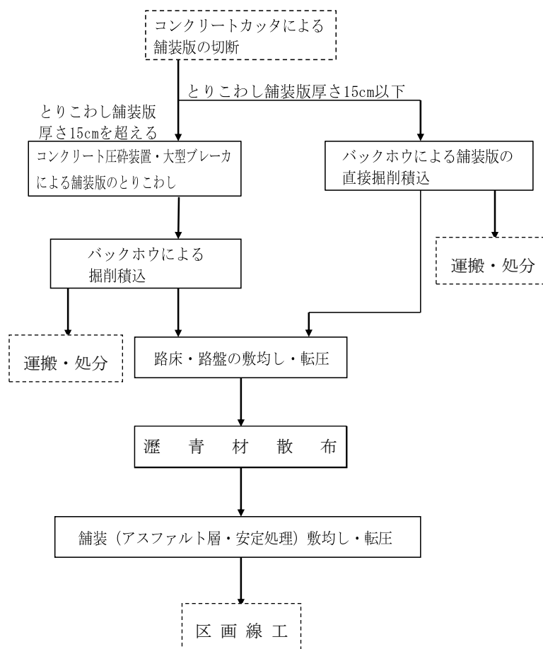
図2-1 施工フロー
