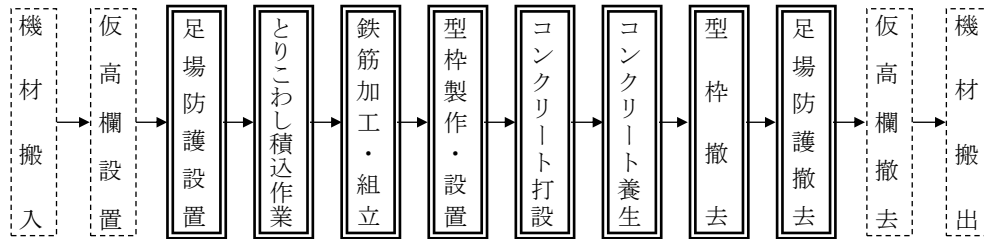
図2-1 施工フロー
