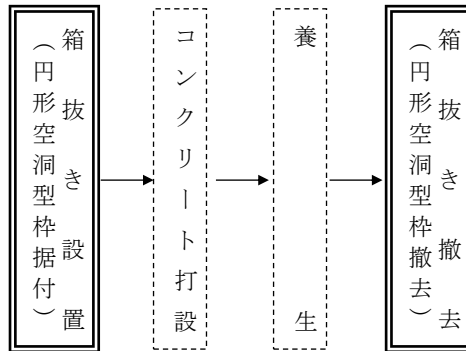
図2-1 施工フロー
