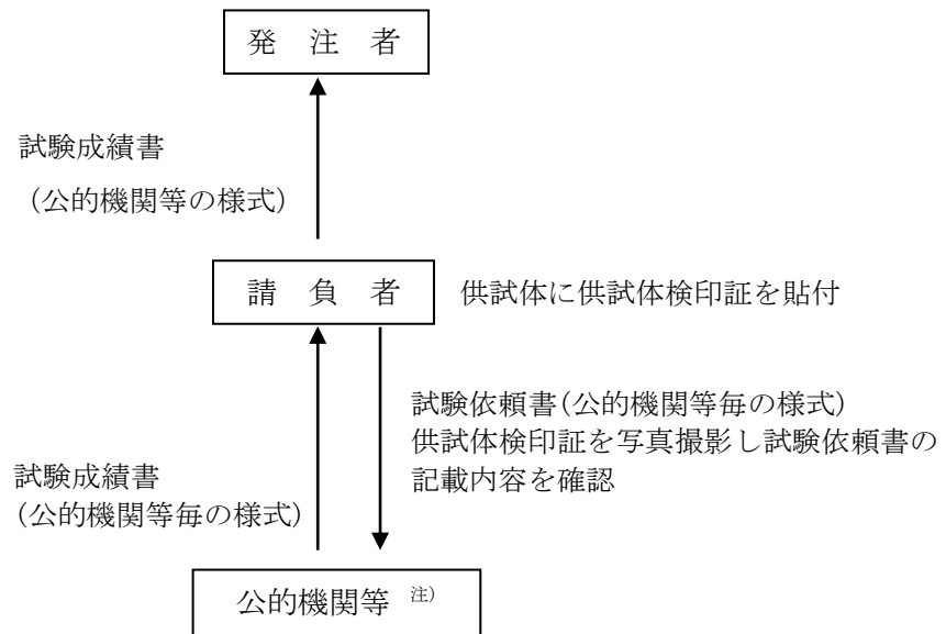
図 11-2 公的機関等での材料試験
