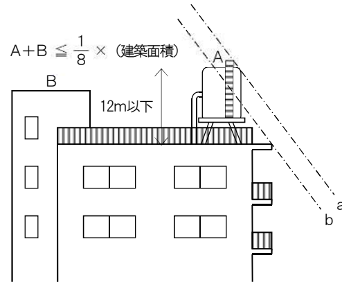
【図2】高架水槽
