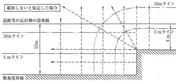
④ 敷地境界線の形状が変化し、発散方向が交錯する場合
