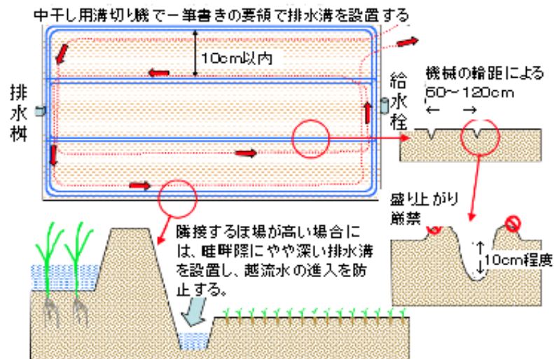
図7 排水溝設置の留意点
