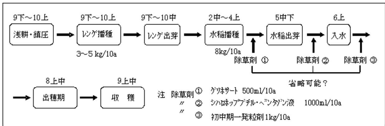
図48 レンゲ立毛中不耕起V溝直播栽培の栽培体系
