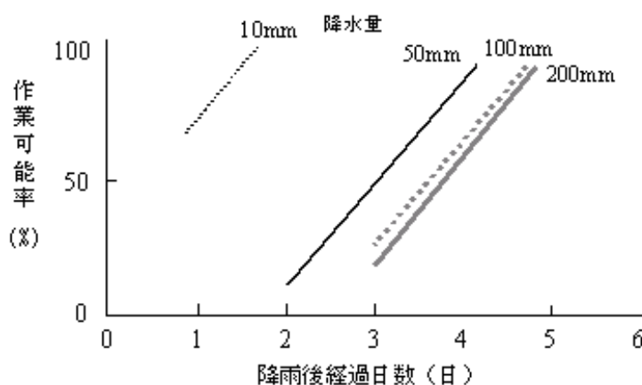
図 19 作業予定前日の降水量と作業可能率の関係
