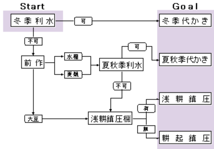
図2 不耕起V溝直播におけるほ場整地法の選択
