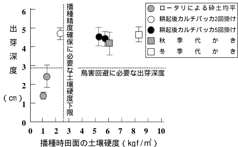
図14 整地の方法が播種時の土壌硬度に及ぼす影響
