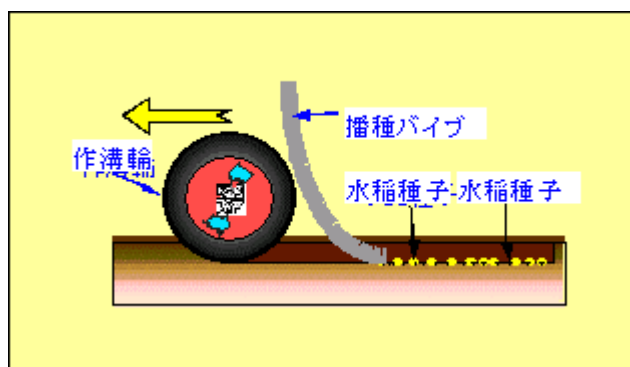
図56 稲麦同時播種の状況
