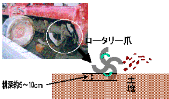
図61 播種前の浅耕による均平
