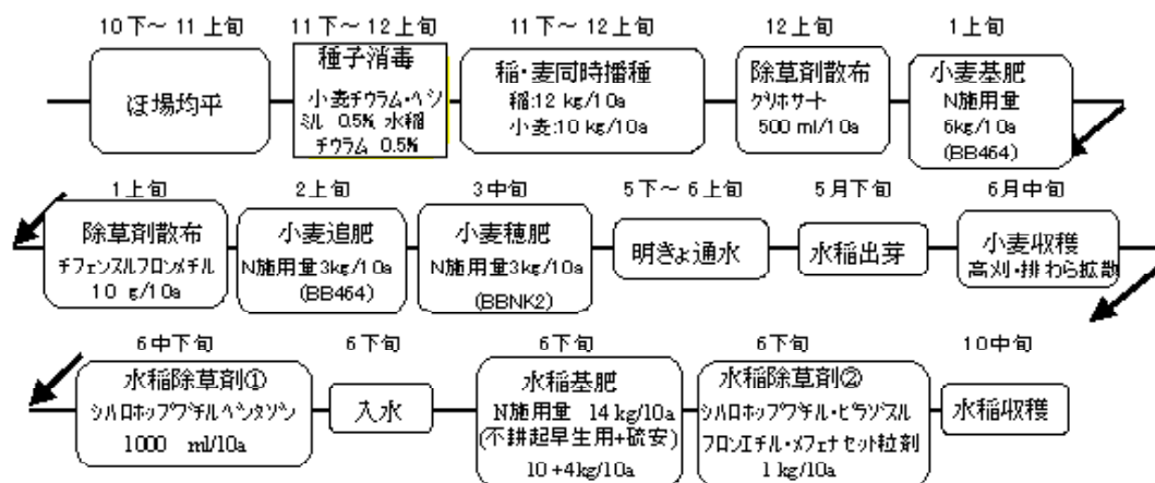
図55 稲麦同時播種栽培技術の体系
