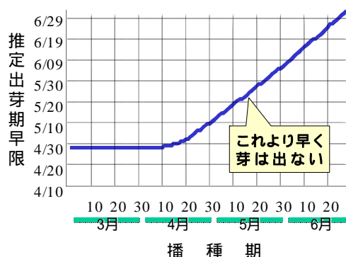
図 35 播種期と出芽早限の関係 (長久手町平年気温によるシミュレーション)
