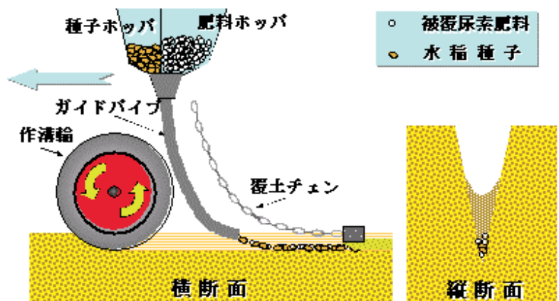
図21 播種様式の模式図
