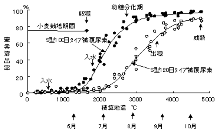
図 51 窒素の溶出パターン
