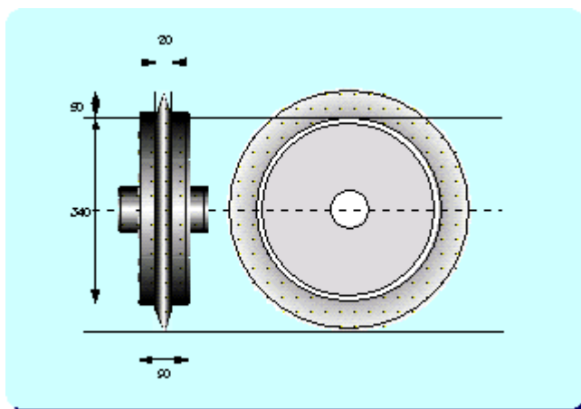
図24 作溝輪の概要
