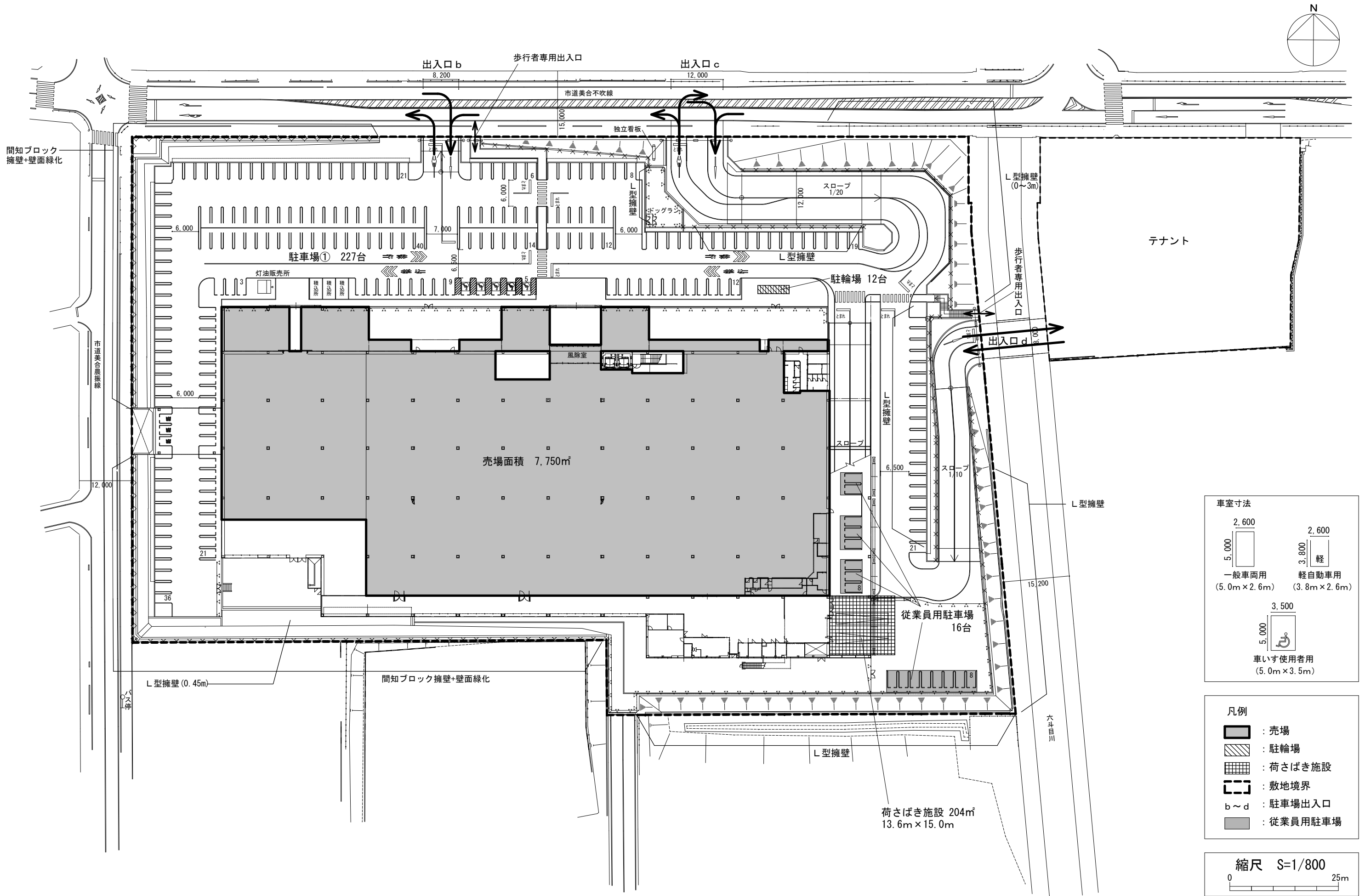
建物配置図兼 1階平面図
