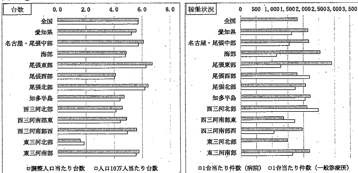
図3-② MRI
