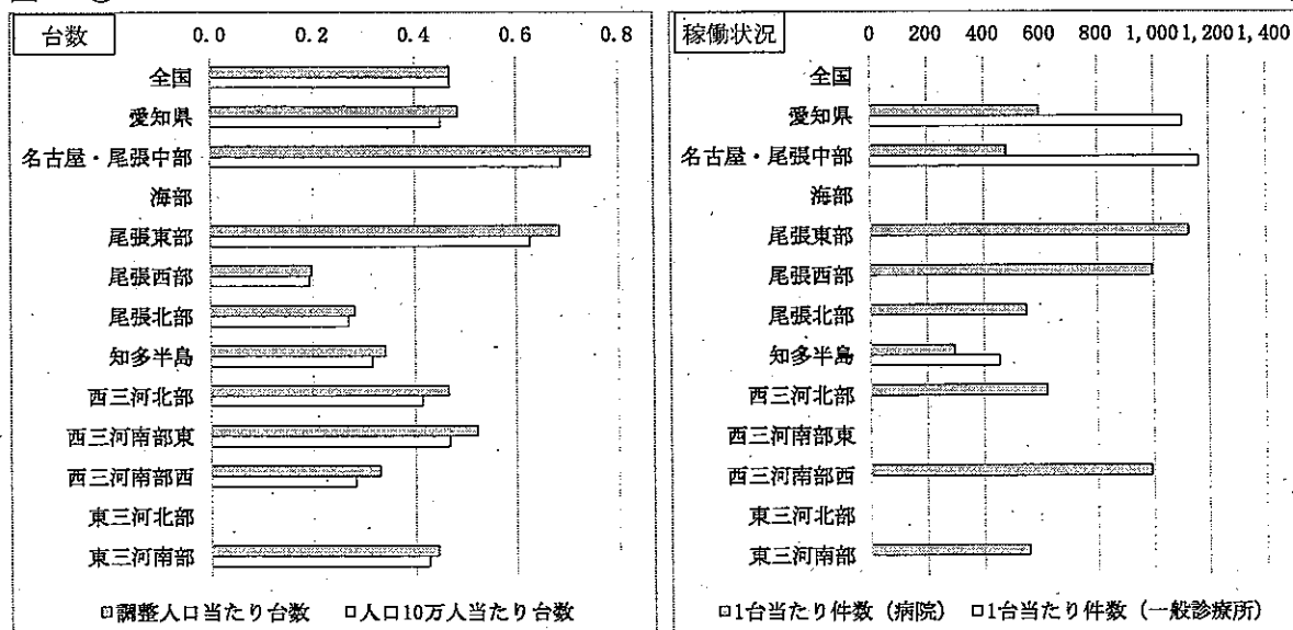
図3-③ PET
