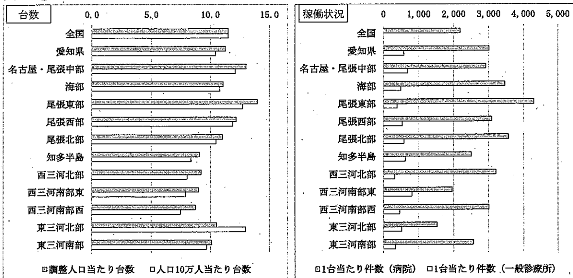
図3-① CT
