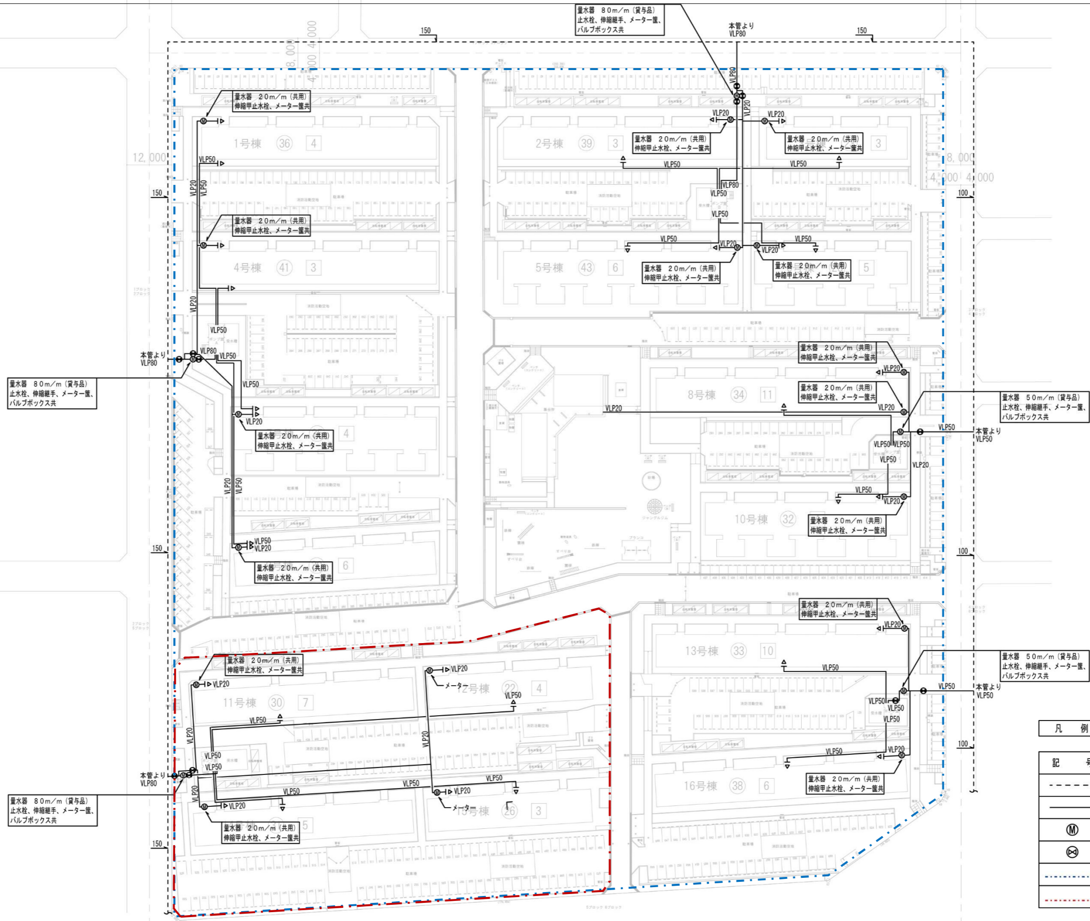
現況給水設備図
