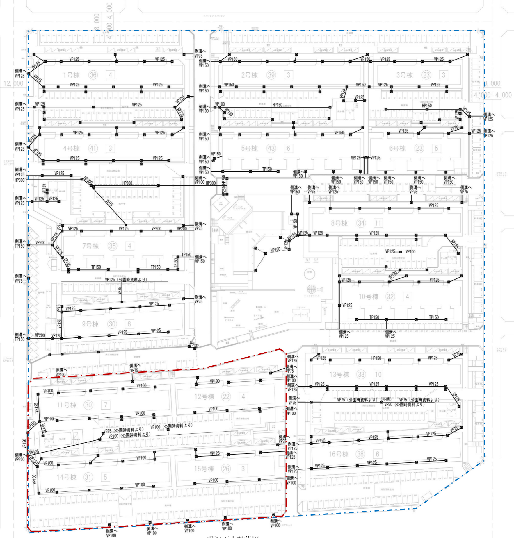
現況雨水設備図
