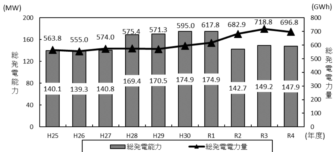
焼却施設におけるごみ発電の状況
