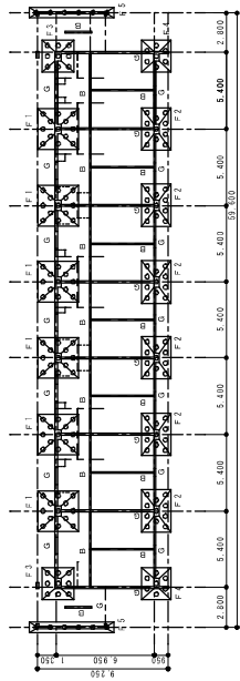
新本館棟(1・2) 基礎平面 基礎柱間 (1-A)-(2)-C-1) 2F 3F 28F 1:200
