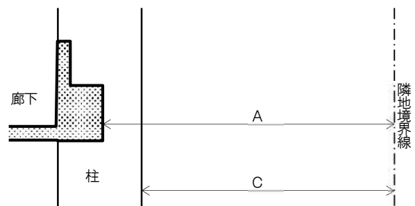
梁がスラブの上にある場合
