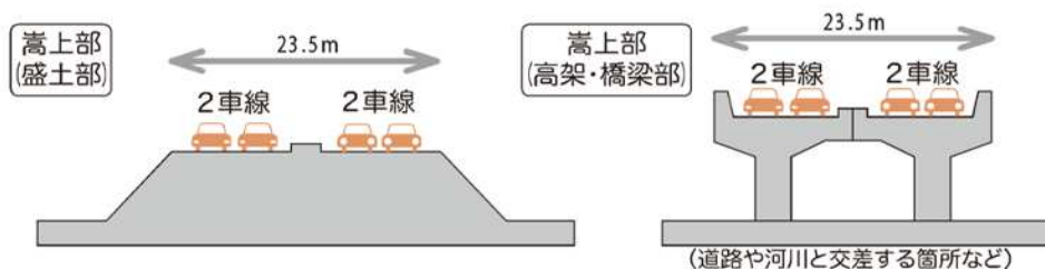
【横断図】
