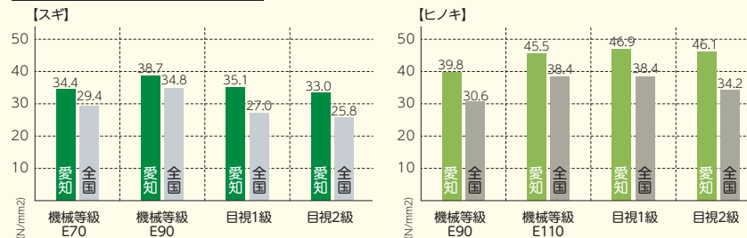
愛知県産スギ・ヒノキ基準強度(曲げ) ※単位 N/mm 2 ※愛知県産材利用の手引き(H29.3発行)より
