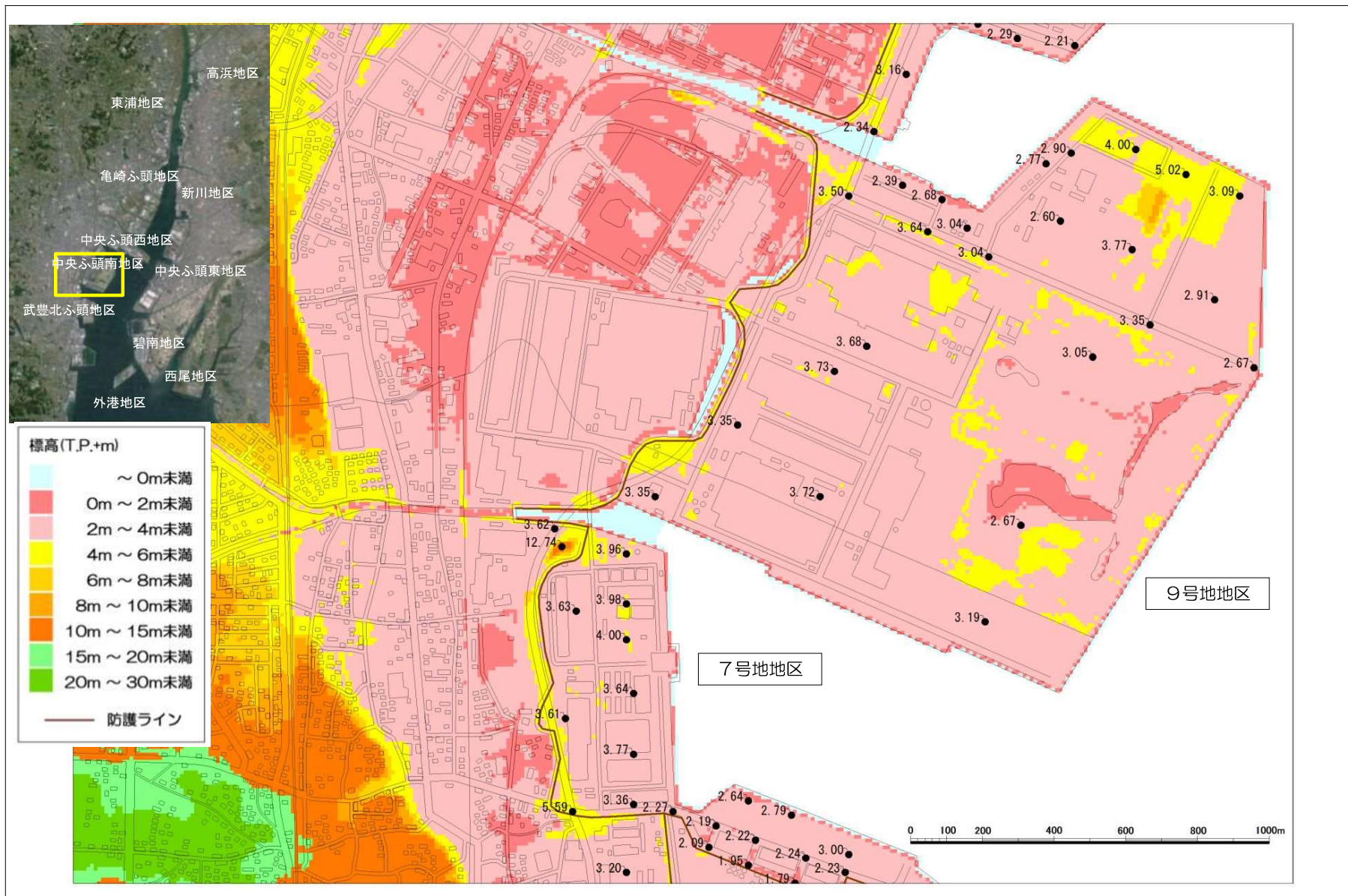
【標高図①】衣浦港 9号地地区・7号地地区(半田市・武豊町)
