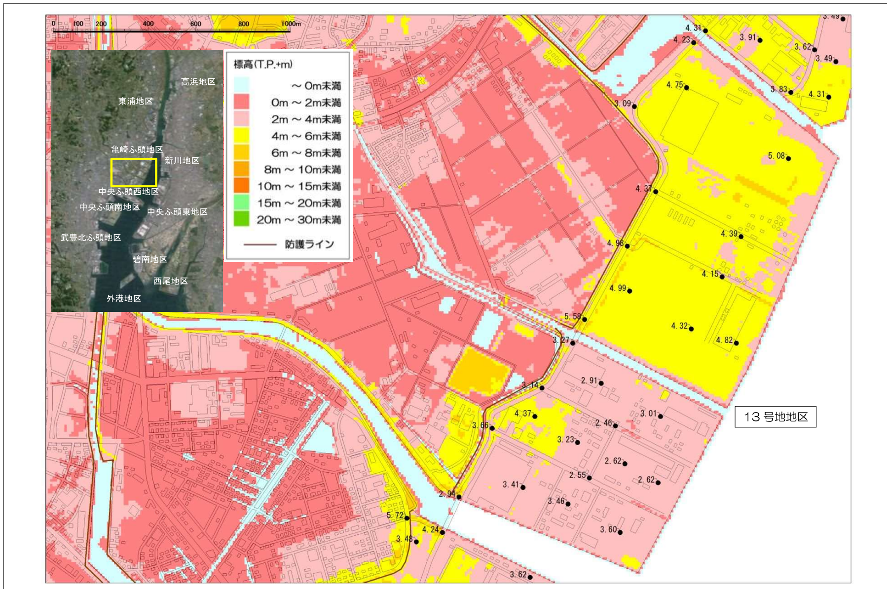
【標高図⑨】衣浦港 13号地地区(半田市)
