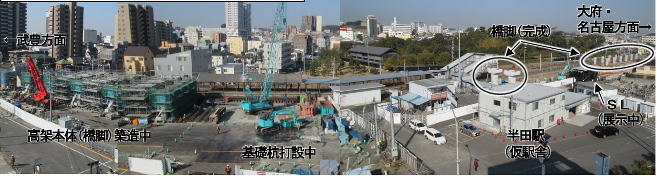
高架本体構造物の築造が進む駅周辺の整備状況
