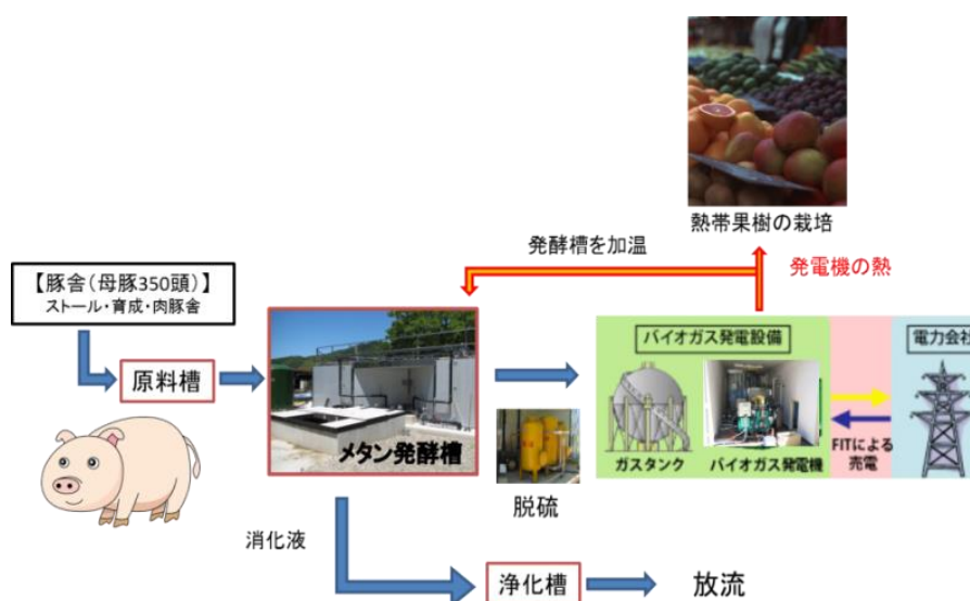
バイオガス発電システム イメージ図
